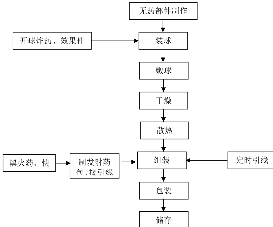
图 2.4-4 礼花类(小礼花)产品生产工艺流程图
