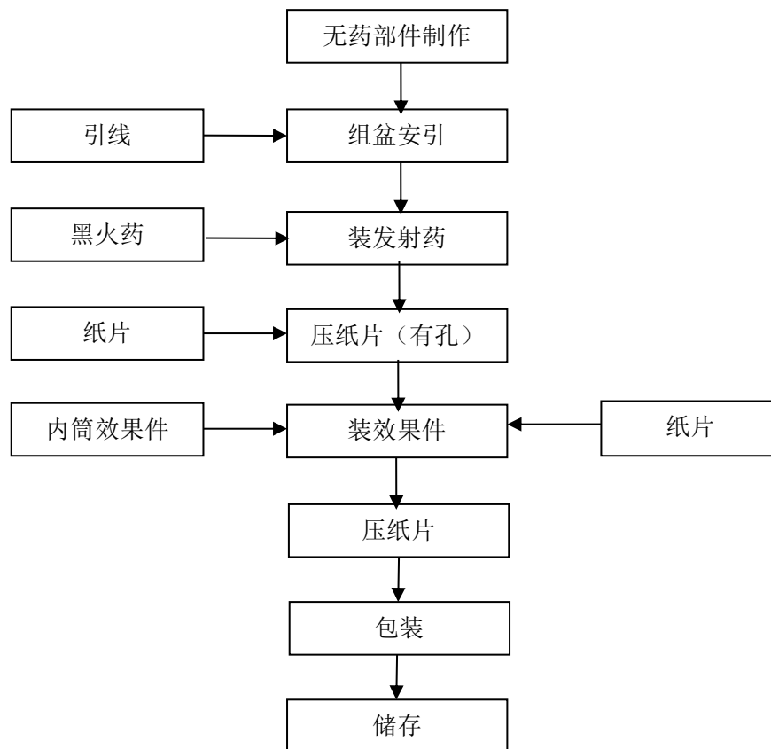
图 2.4-3 组合烟花生产工艺流程图
