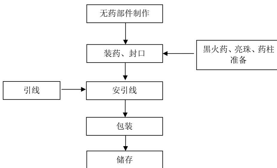
图 2.4-5 喷花类产品生产流程图
