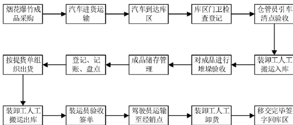
图 2.8 烟花爆竹产品经营工艺流程图
