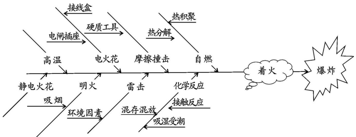
图 3.3-1 烟花爆竹引爆的因果分析图
