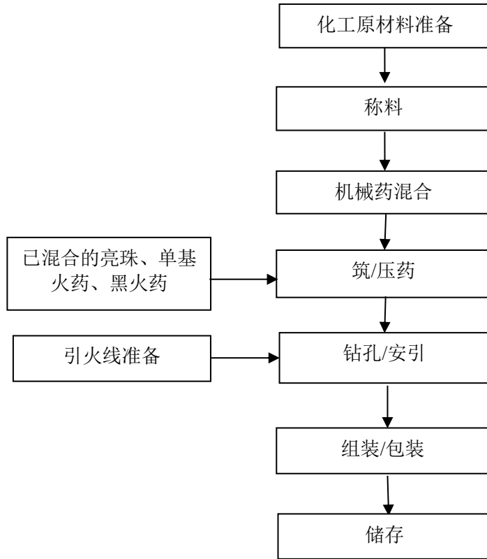
图 2.4-2 喷花类产品生产工艺流程图
