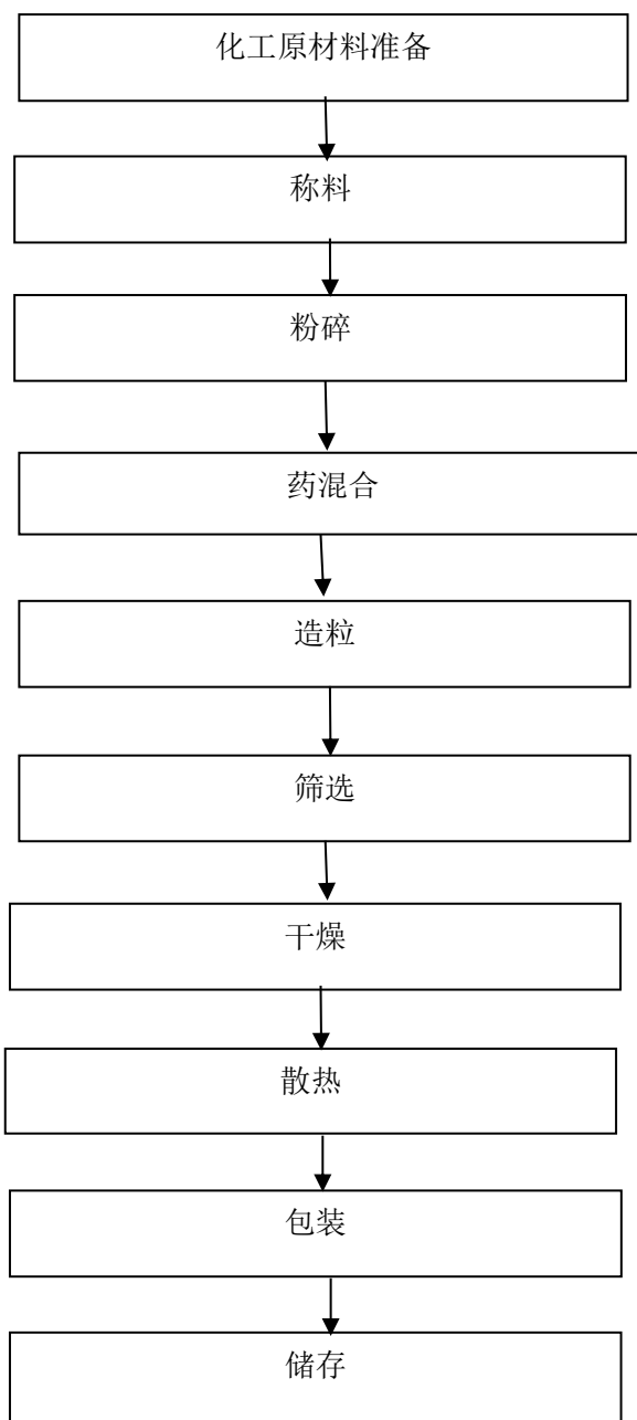
图 2.4-1 亮珠生产工艺流程图
