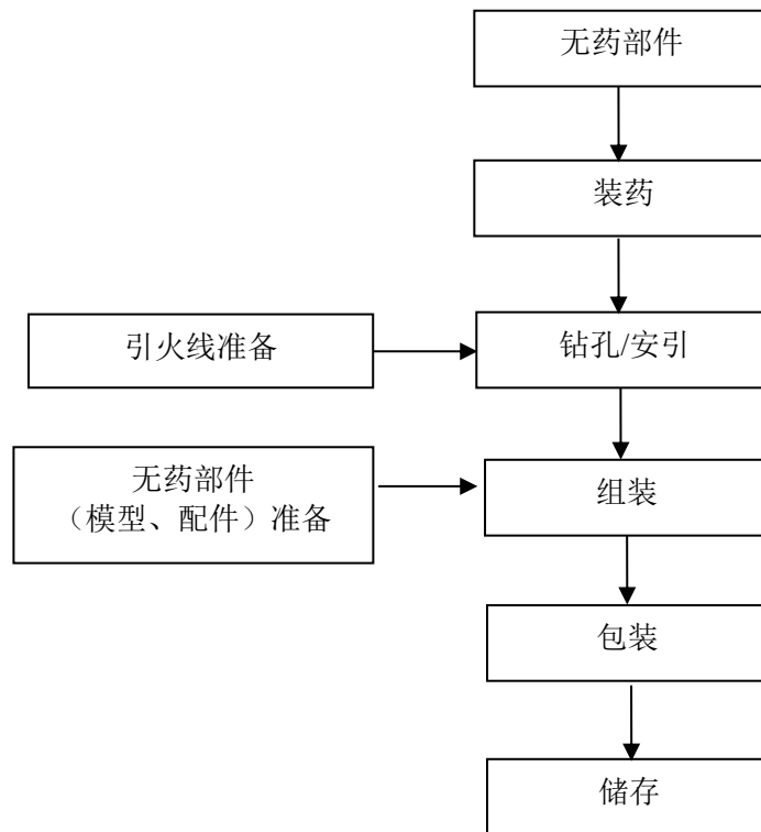
图 2.4-3 玩具类（造型玩具）产品生产工艺流程图
