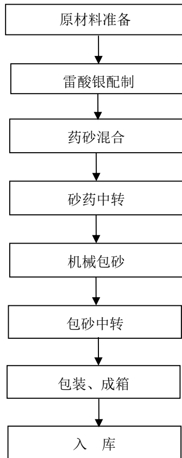
图 2.4-4 玩具类（摩擦型/砂炮）产品生产工艺流程图
