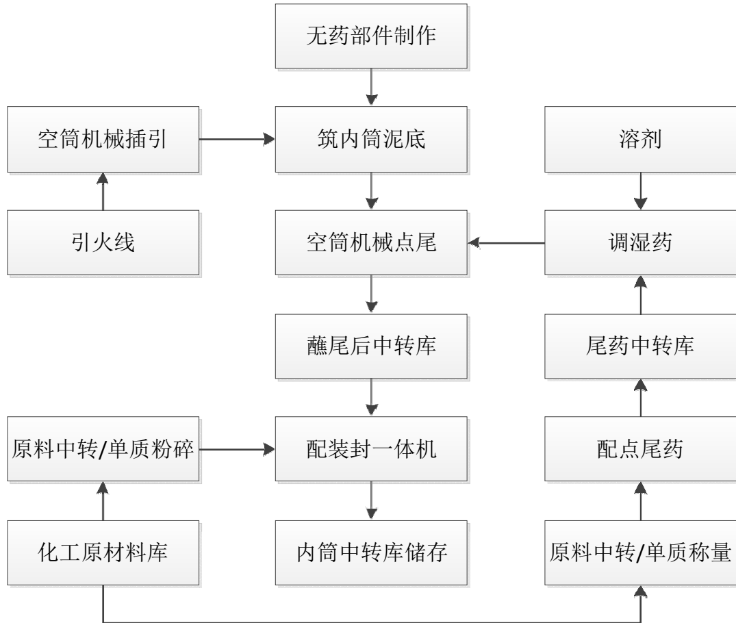
图 2.3-1 内筒制作生产工艺流程图（金泰分厂）
