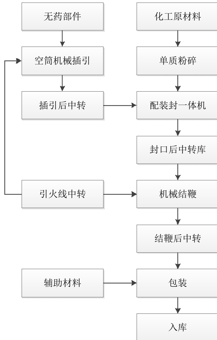
图 2.3-3 爆竹类生产工艺流程图（金瑞分厂）
