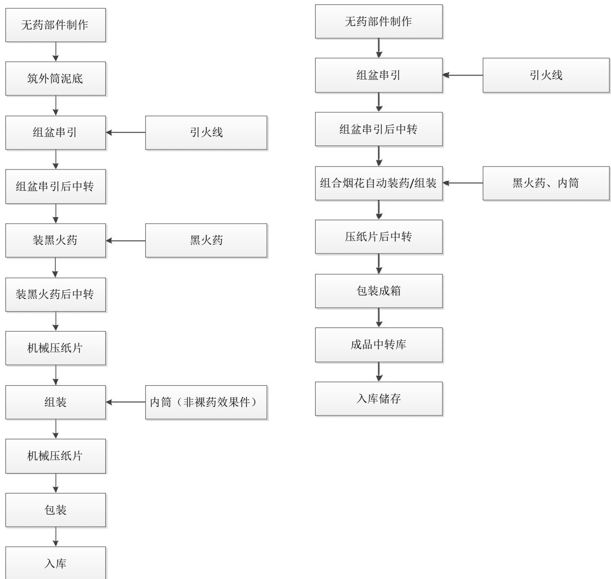
图 2.3-2 组合烟花类生产工艺流程图（金泰分厂）
