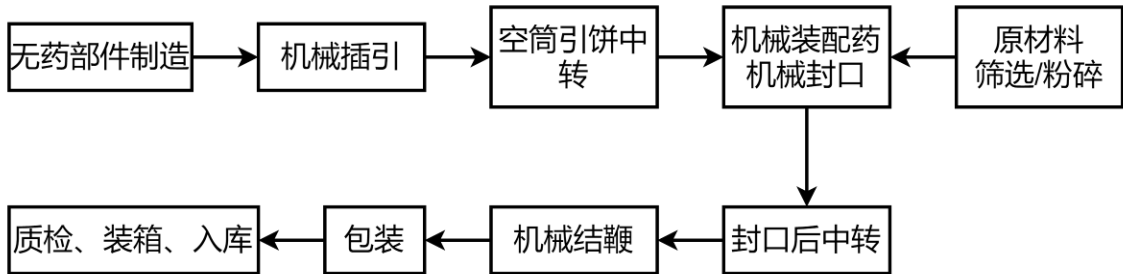
图 2-2：爆竹生产（插引）工艺流程
