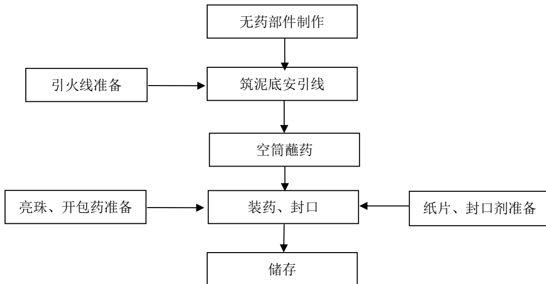
图 2.6-2 效果内筒生产工艺流程图
