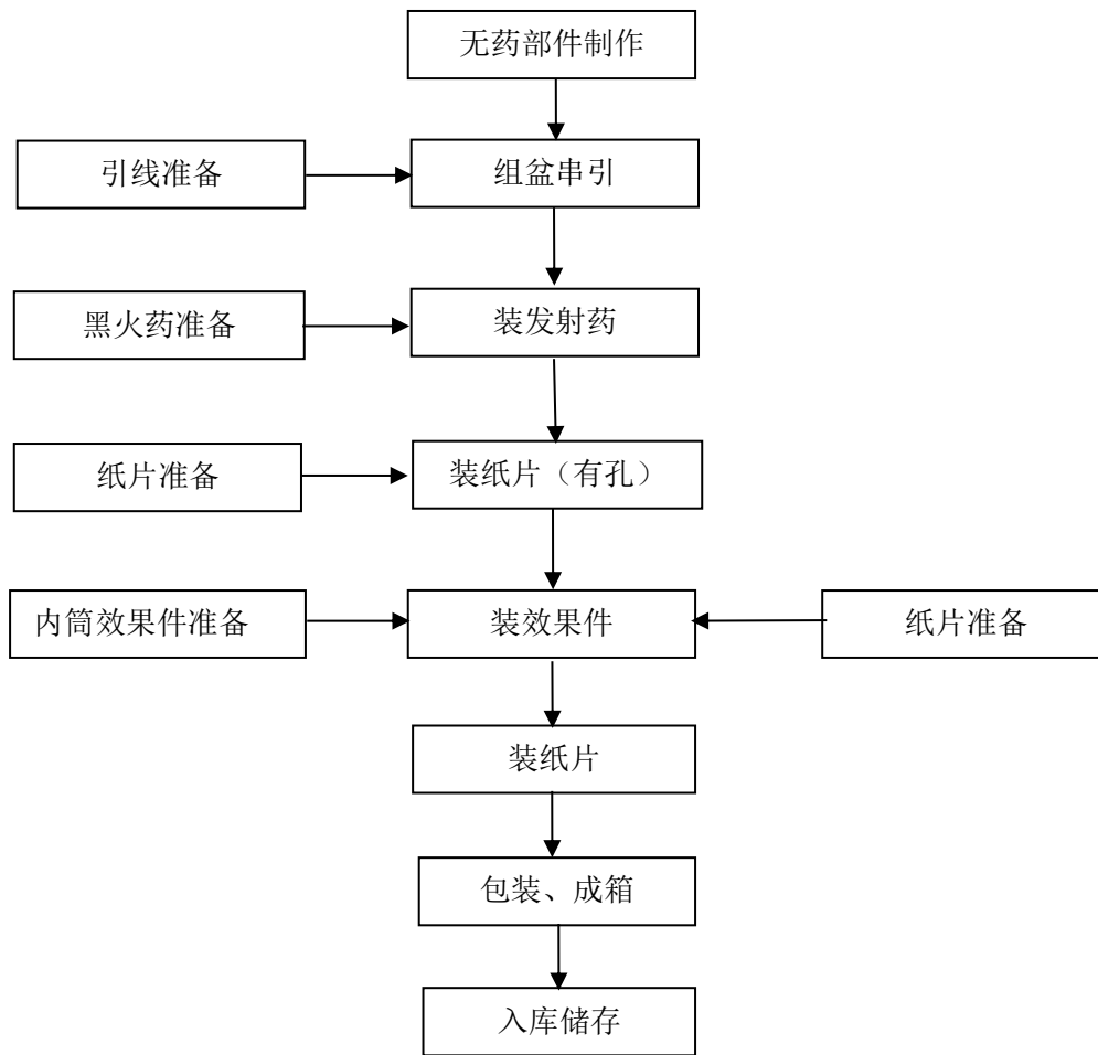
图 2.6-3 组合烟花类产品生产工艺流程图
