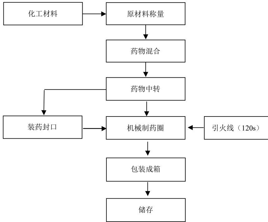
图 2-2：旋转类（花环）生产工艺流程图
