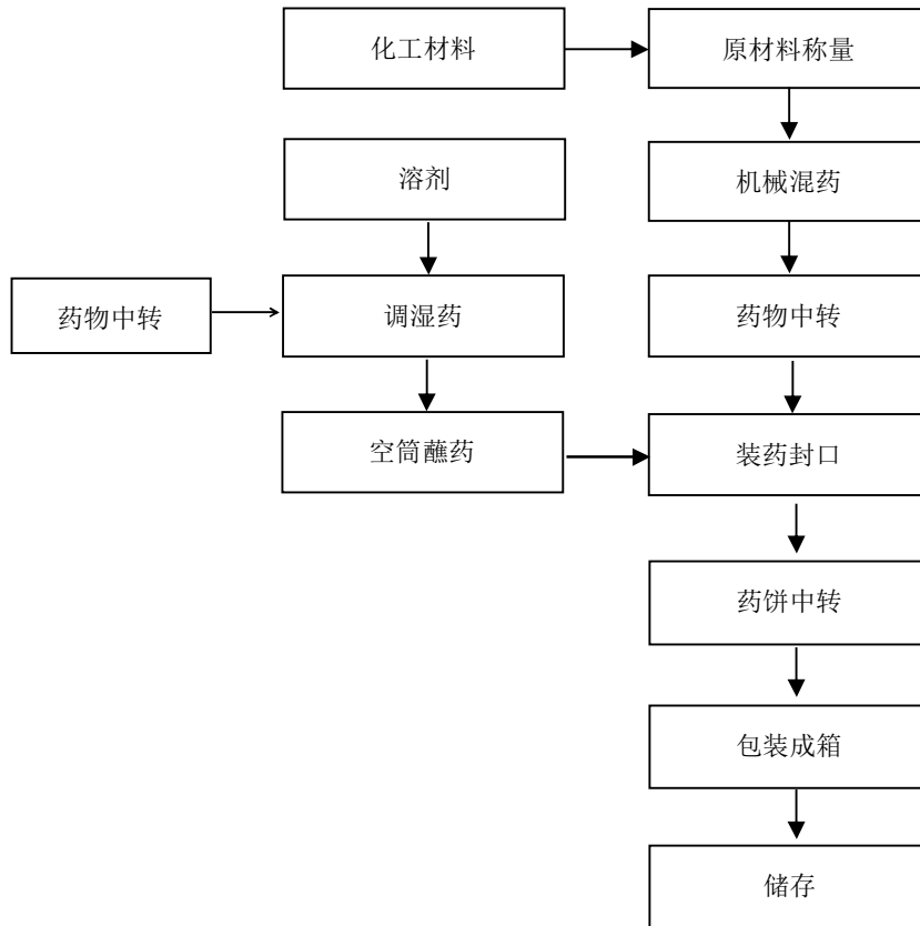
图 2-3：旋转玩具类（线香型-晨光花）生产工艺流程图
