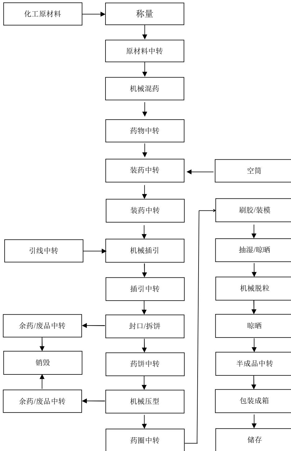
图 2-1：旋转类（彩菊）生产工艺流程图
