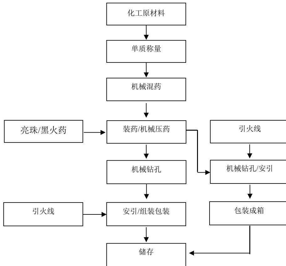
图 2-2：升空类（旋转升空烟花）生产工艺流程图
