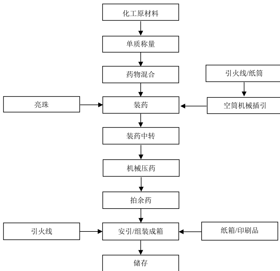
图 2-1：升空类（火箭）生产工艺流程图
