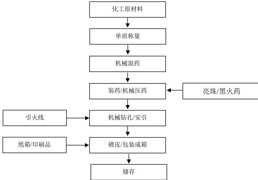
图 2-4：旋转类（大地花开）生产工艺流程图
