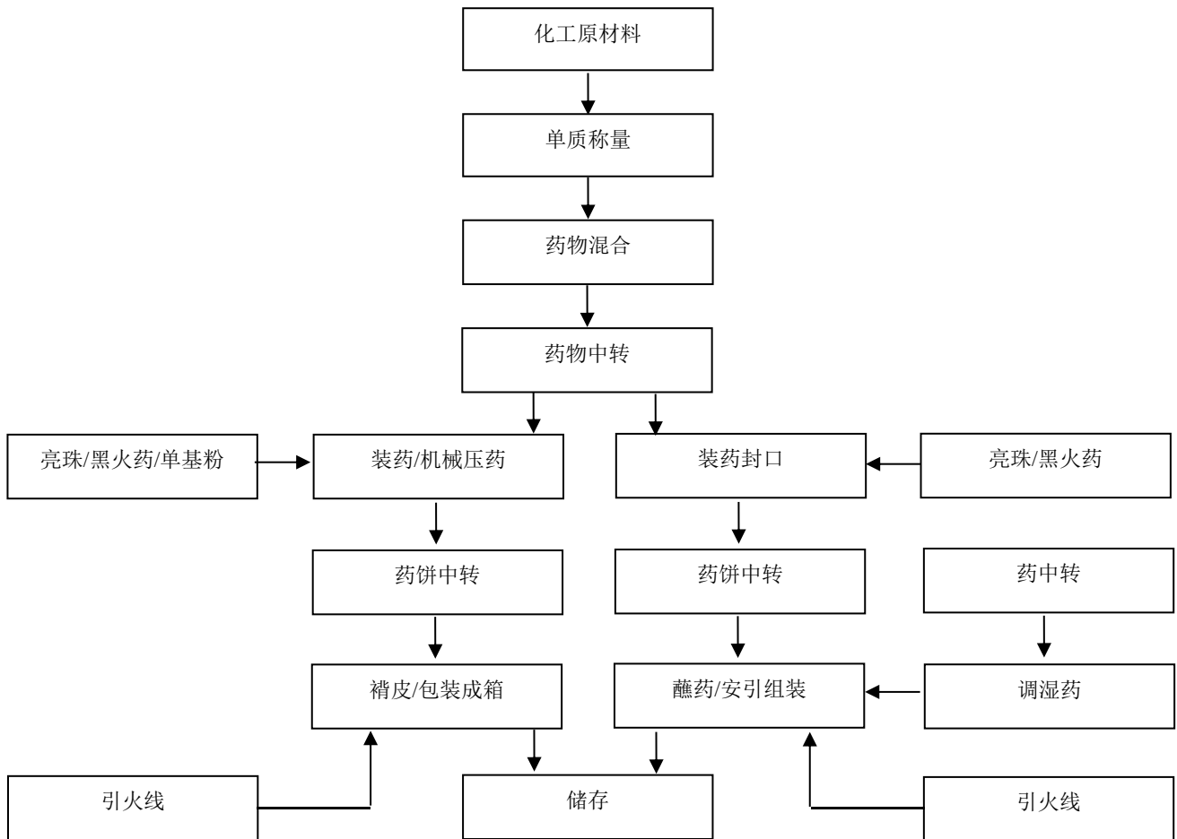
图 2-3：喷花类生产工艺流程图
