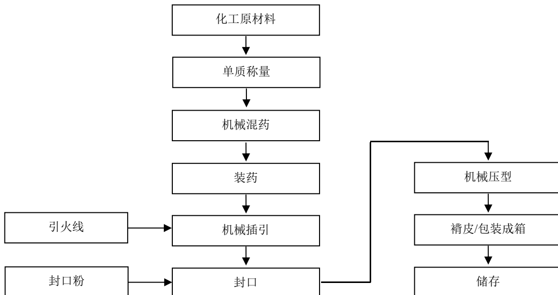
图 2-5：旋转类（茶花香）生产工艺流程图
