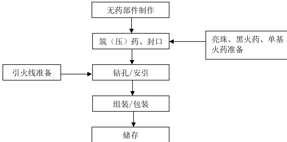
图 2.4-3 喷花类产品生产工艺流程图
