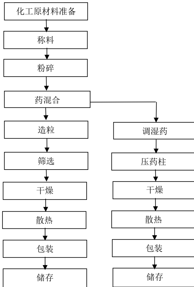
图 2.4-1 亮珠、药柱生产工艺流程图
