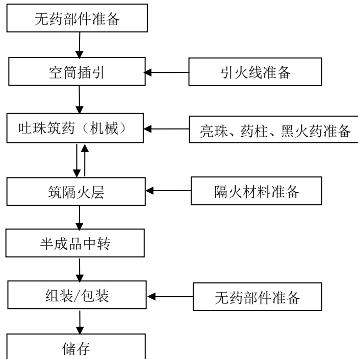
图 2.4-2 吐珠类产品生产工艺流程图
