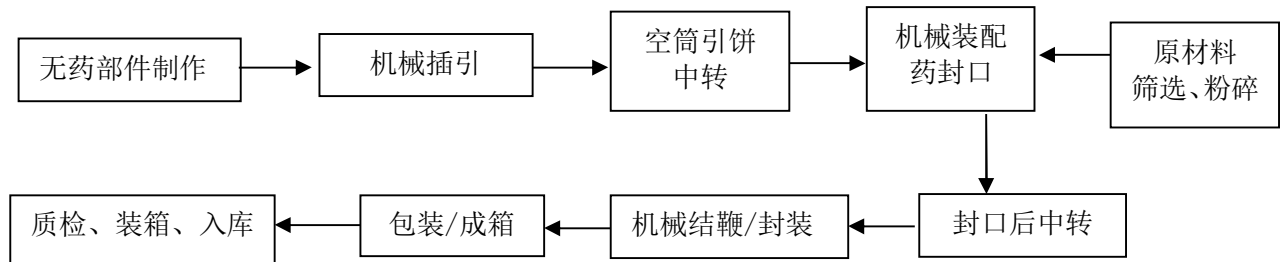
图 2-1 爆竹生产（插引）工艺流程图
