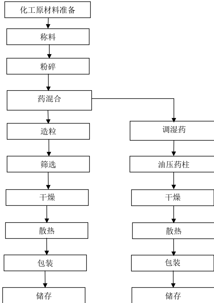
图 2.4-1 亮珠、药柱生产工艺流程图
