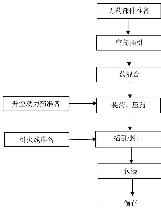
图 2.4-4 升空类（小型火箭）产品生产工艺流程图
