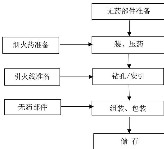
图 2.4-5 升空类（旋转升空烟花）产品生产工艺流程图
