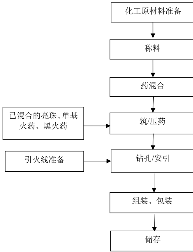
图 2.4-2 喷花类产品生产工艺流程图
