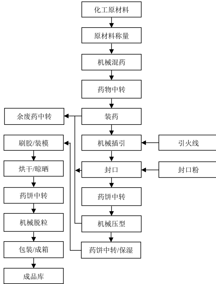
图 2-1：旋转类（彩菊）生产工艺流程图
