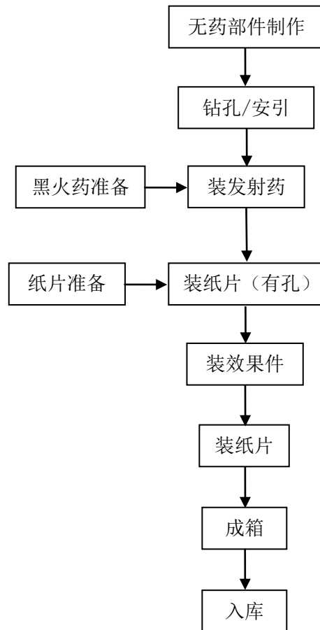
图 2.6-5 礼花类（圆柱/药粒/药柱型小礼花）生产工艺流程图
