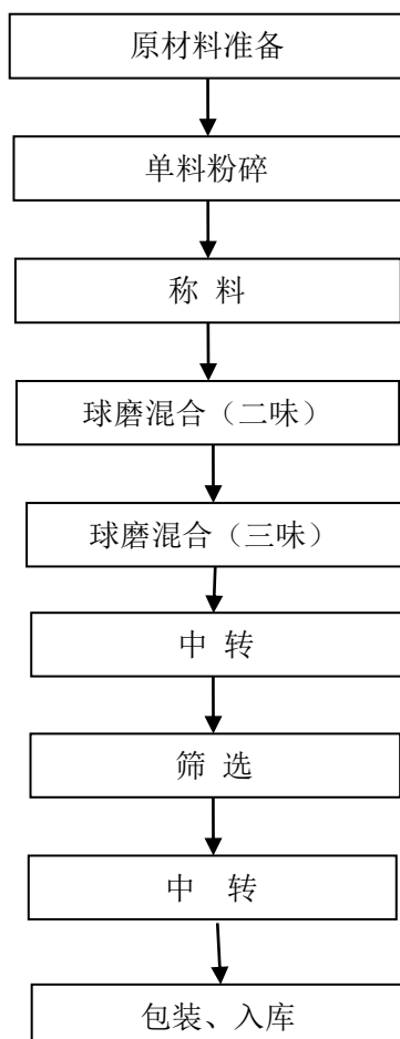
图 2.4-1 黑火药(粉状)产品生产工艺流程图
