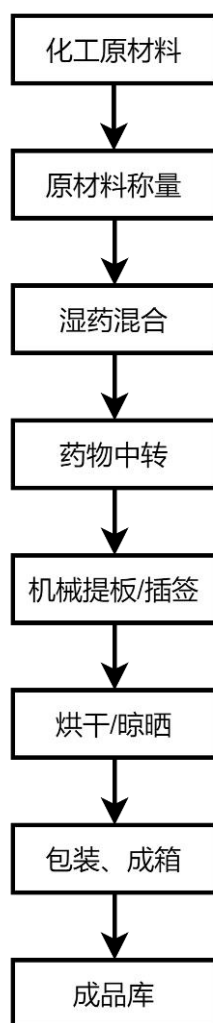
图 2-3: C 级玩具类(线香型)工艺流程
