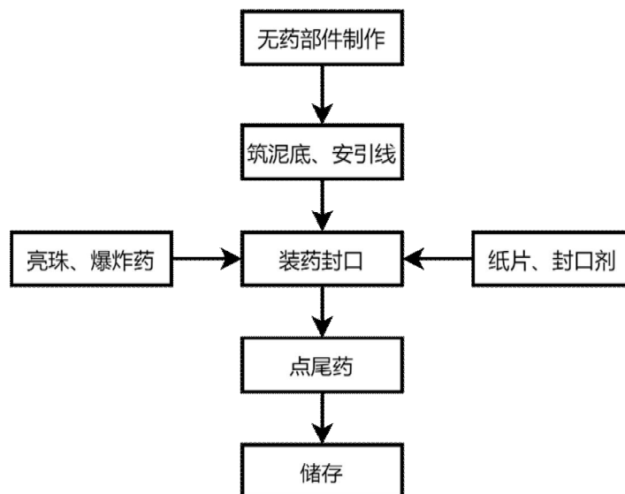
图 2-2：效果内筒工艺流程图
