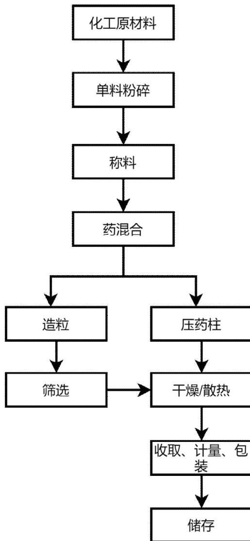
图 2-3：烟火药（亮珠/药柱）工艺流程图
