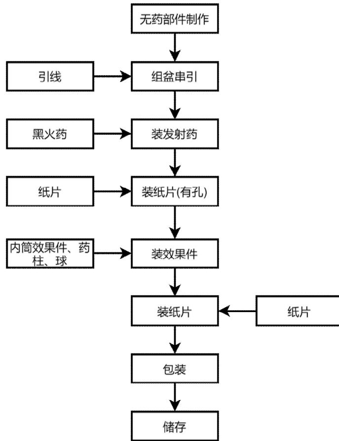
图 2-1：C 级组合烟花类工艺流程图
