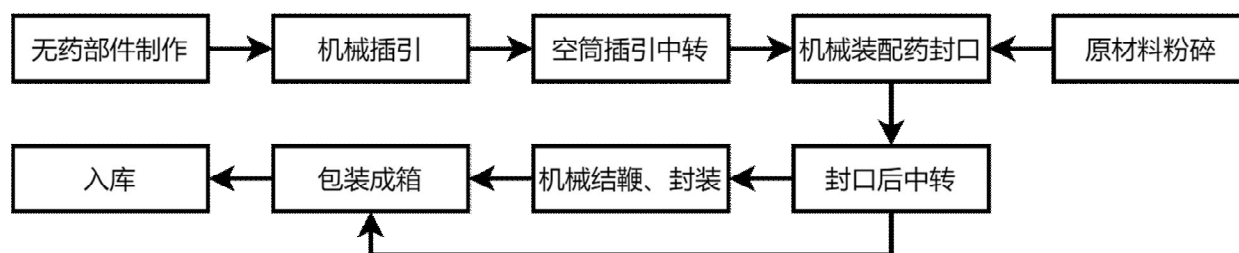
图 2-1: C 级爆竹类(白药炮)工艺流程图
