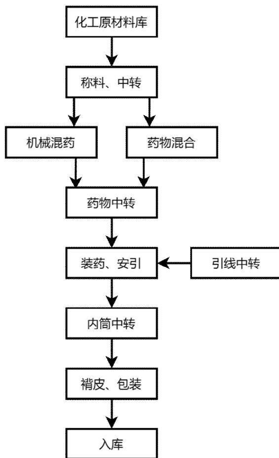
图 2-3：C、D 级玩具类(玩具造型)工艺流程图
