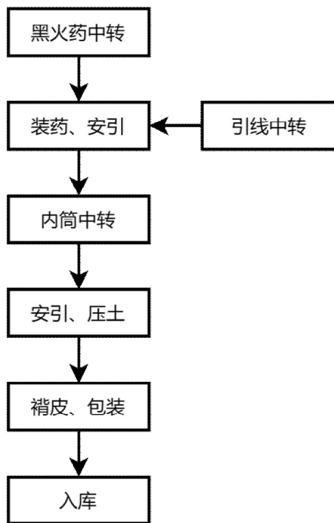
图 2-4：C、D 级玩具类(玩具造型/地雷炮)工艺流程图
