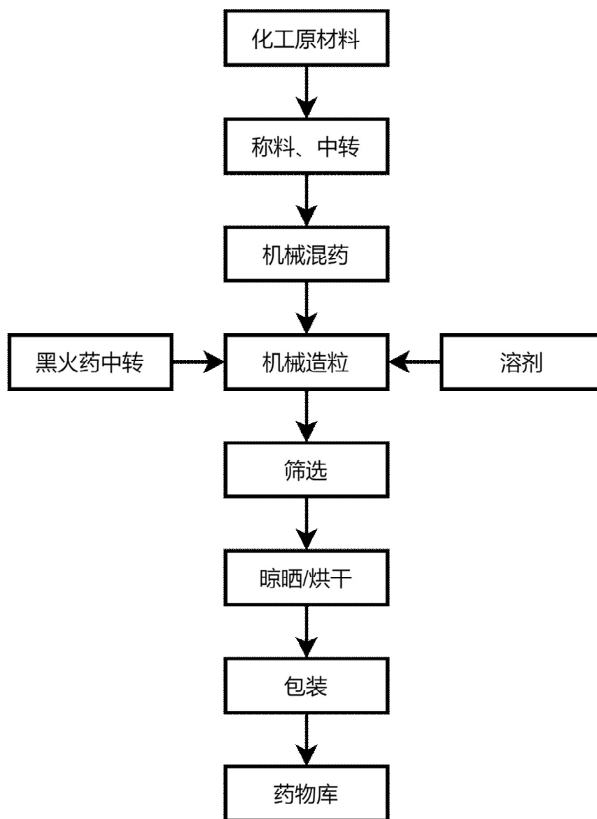
图 2-6：烟花药(仅限亮珠自产自用)工艺流程图
