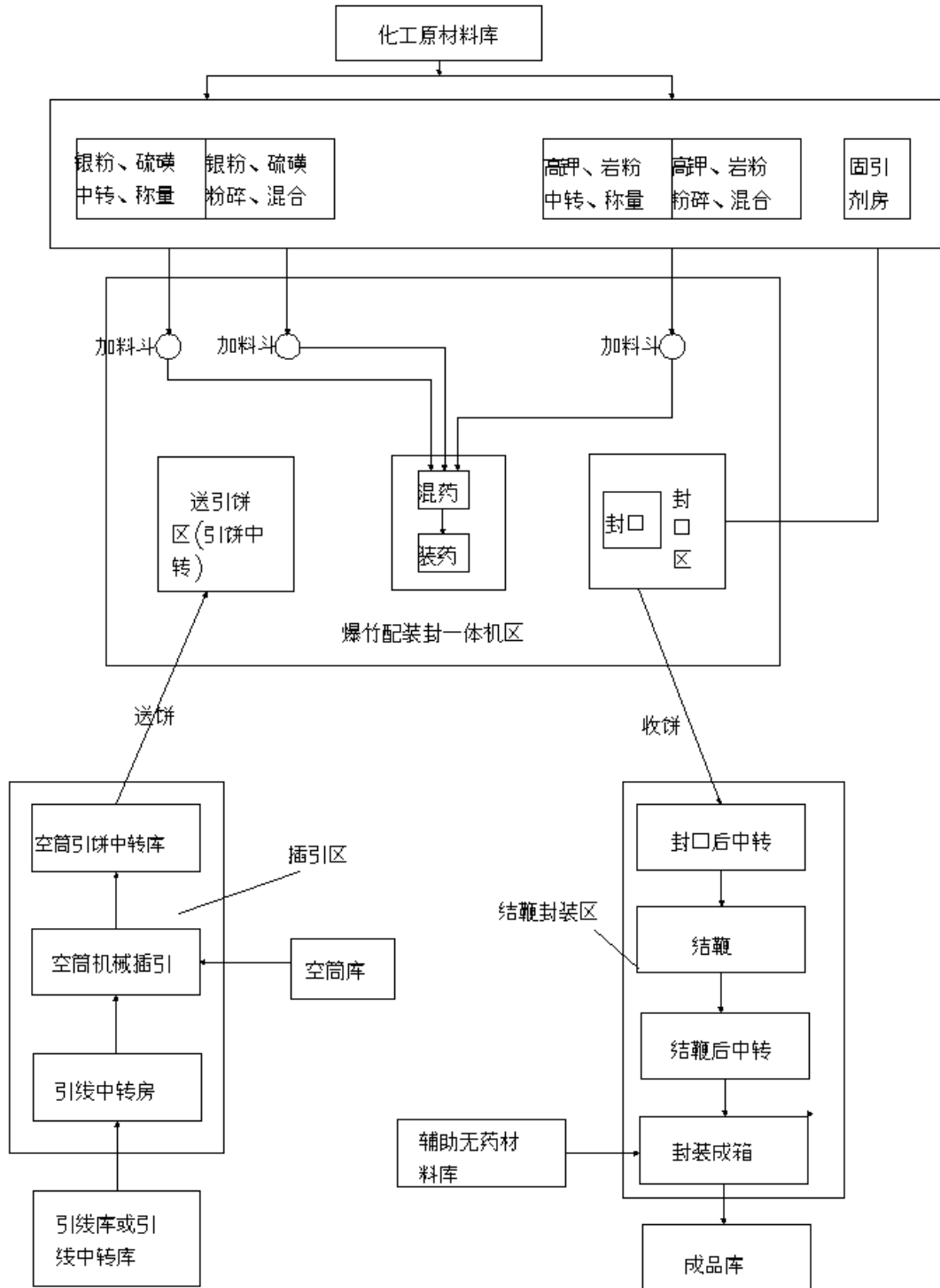
图 2-1：爆竹生产（插引）工艺流程
