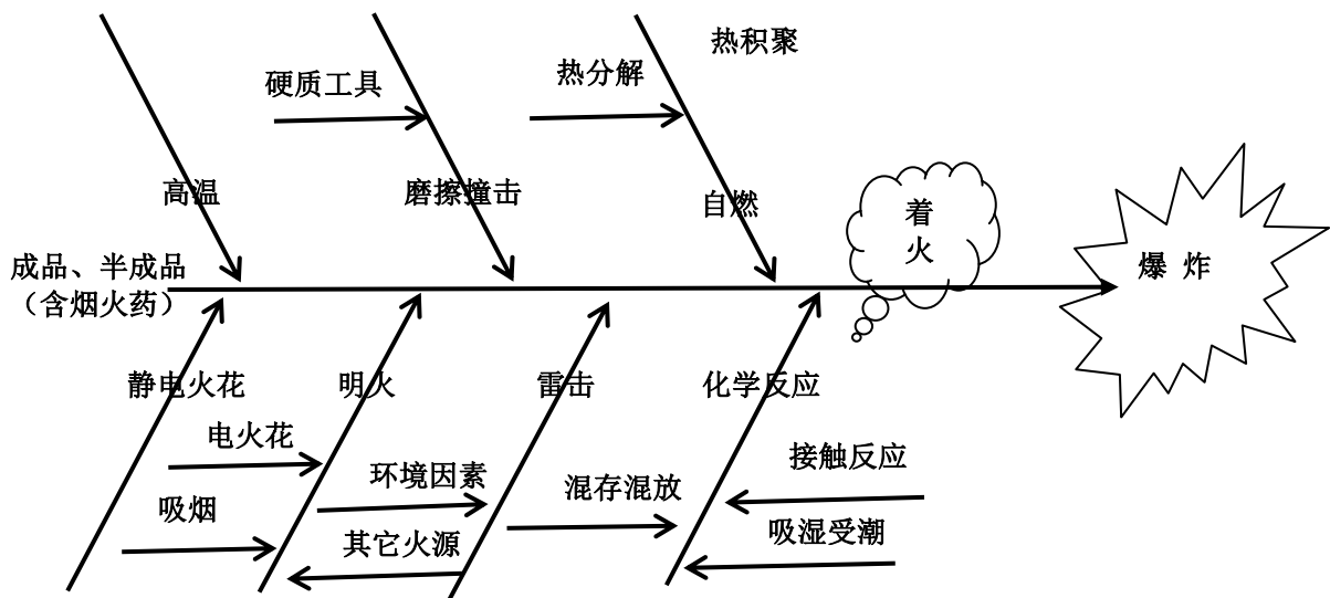
图 3.7-1 仓储场所爆炸的因果分析图
