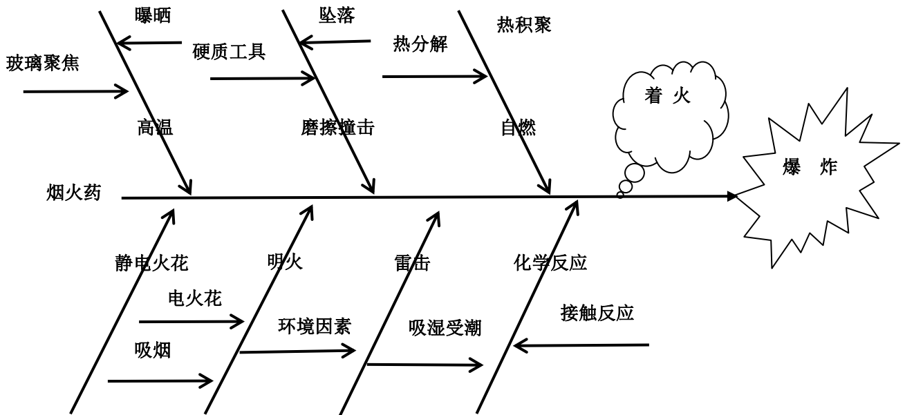
图 3.11-3 黑火药燃烧、爆炸触发条件分析图
