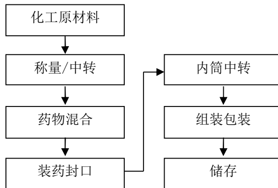
图 2-2：喷花类产品生产工艺流程图
