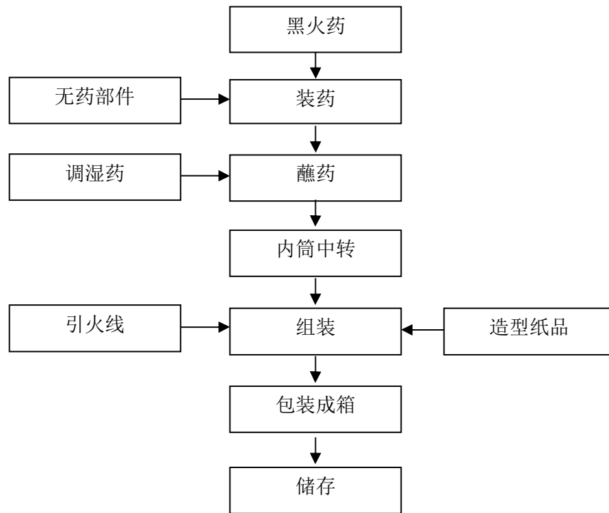
图 2-3：玩具类（玩具造型）产品生产工艺流程图
