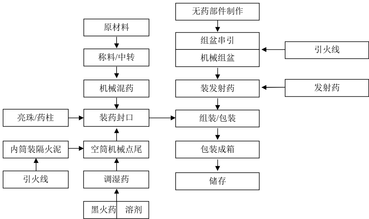
图 2-1：组合烟花类产品生产工艺流程图
