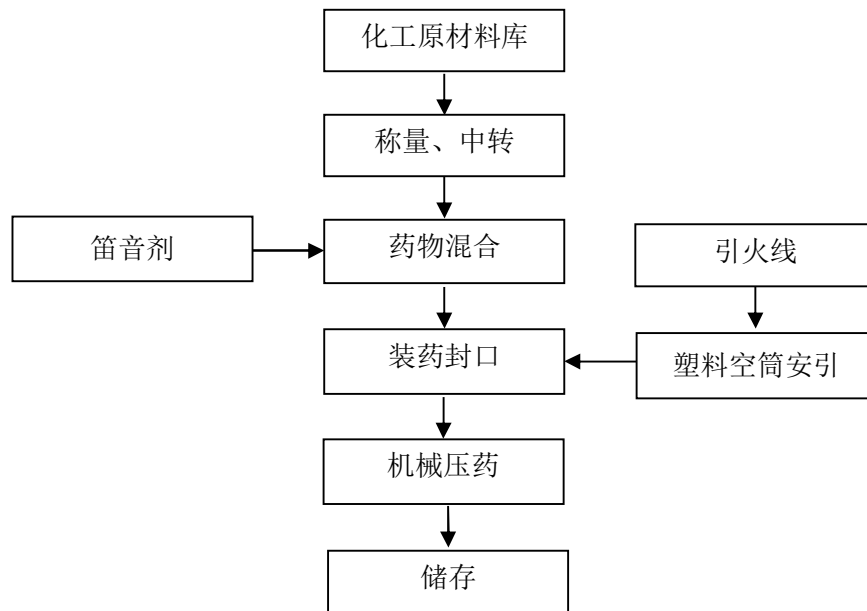
图 2-4：笛音（叫筒）生产工艺流程图
