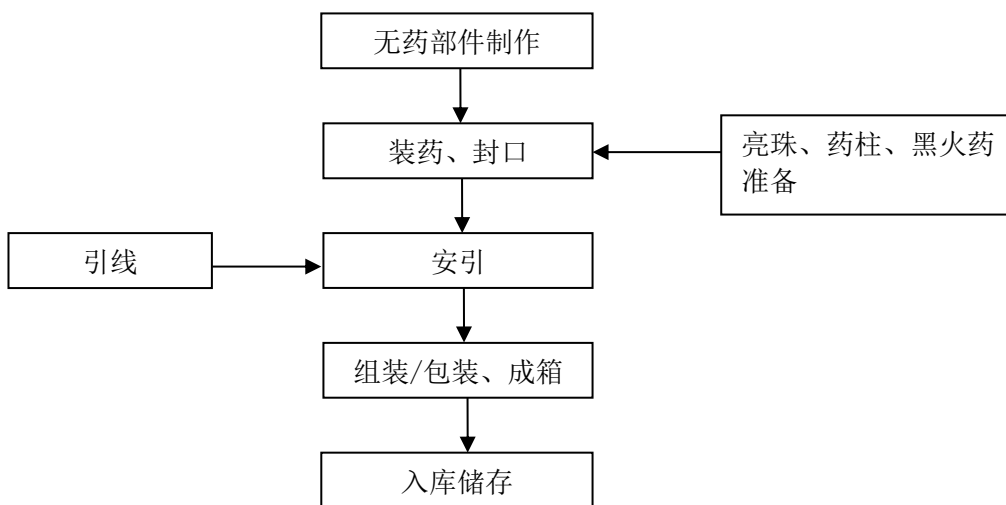
图 2.4-4 喷花类产品生产工艺流程图
