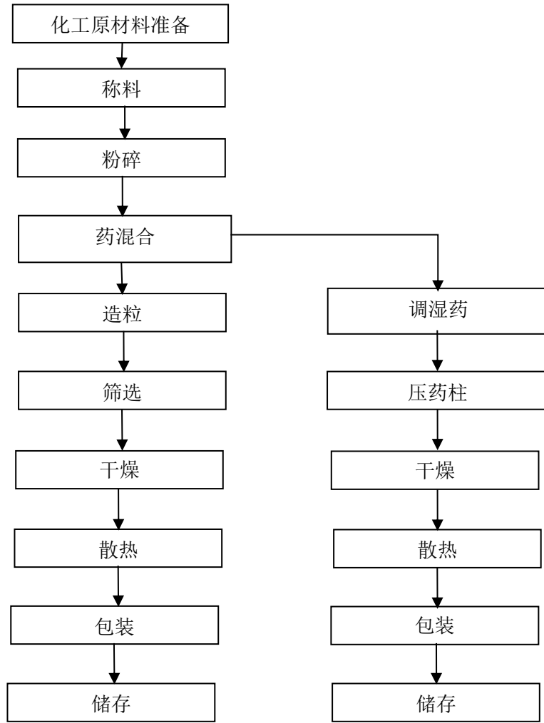
图 2.6-1 亮珠、药柱生产工艺流程图
