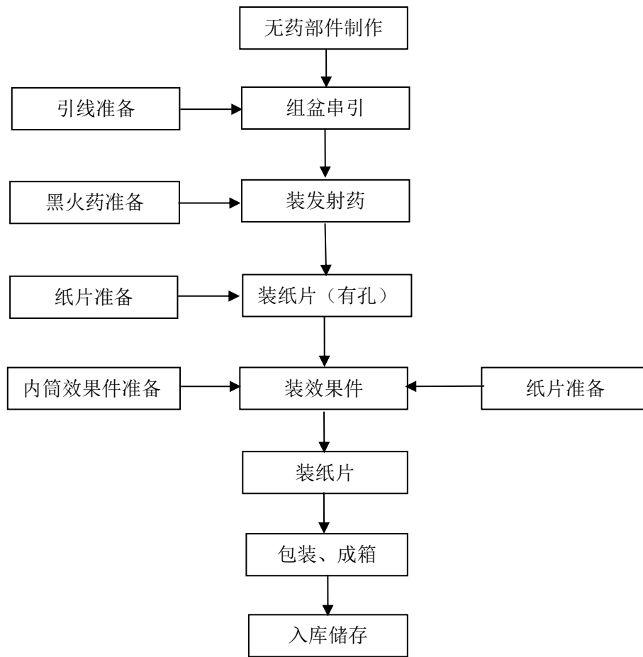
图 2.6-3 组合烟花类产品生产工艺流程图
