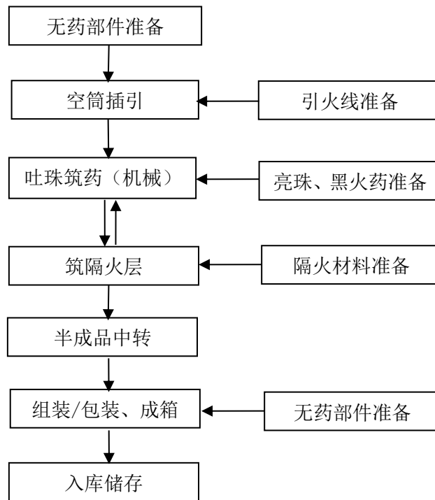
图 2.6-5 吐珠类产品生产工艺流程图
