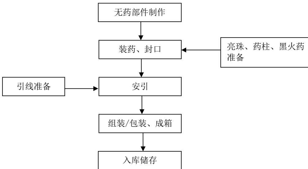
图 2.6-4 喷花类产品生产工艺流程图
