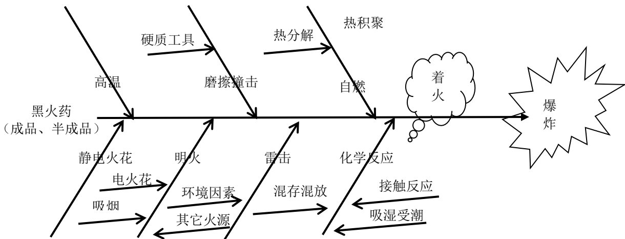
图 3.7-1 仓储场所爆炸的因果分析图
