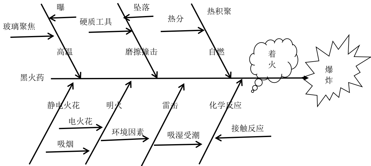
图 3.11-3 黑火药燃烧、爆炸触发条件分析图
