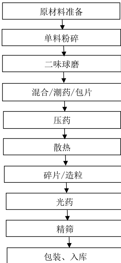
图 2.4-2 黑火药（粒状）产品生产工艺流程图
