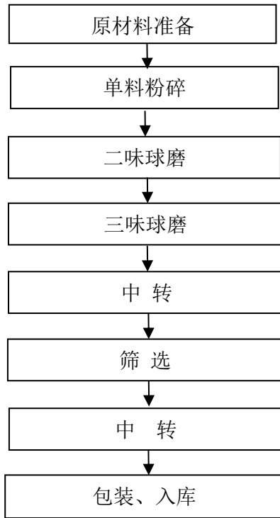
图 2.4-1 黑火药（粉状）产品生产工艺流程图
