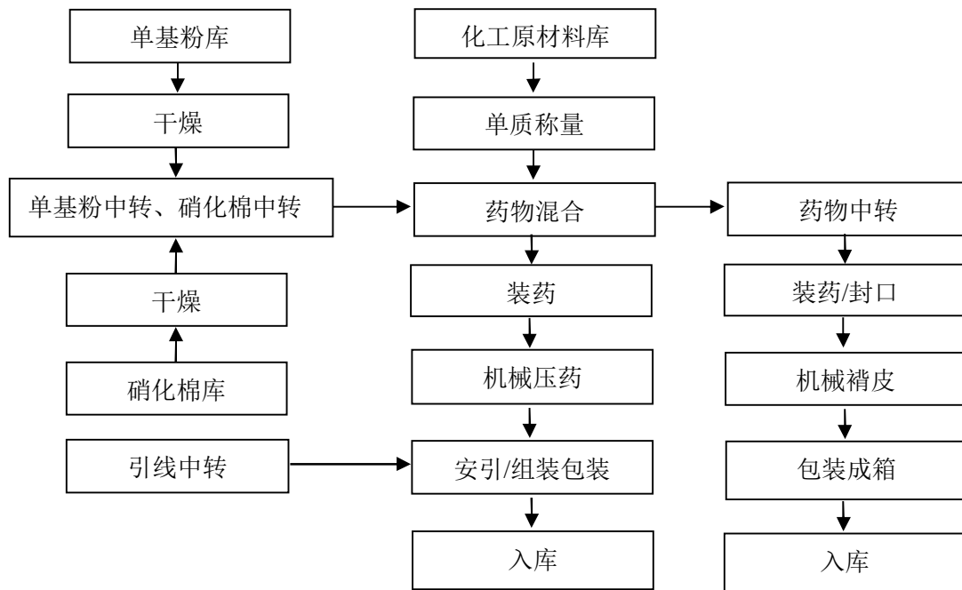
图 2.3-1：喷花类生产工艺流程图
