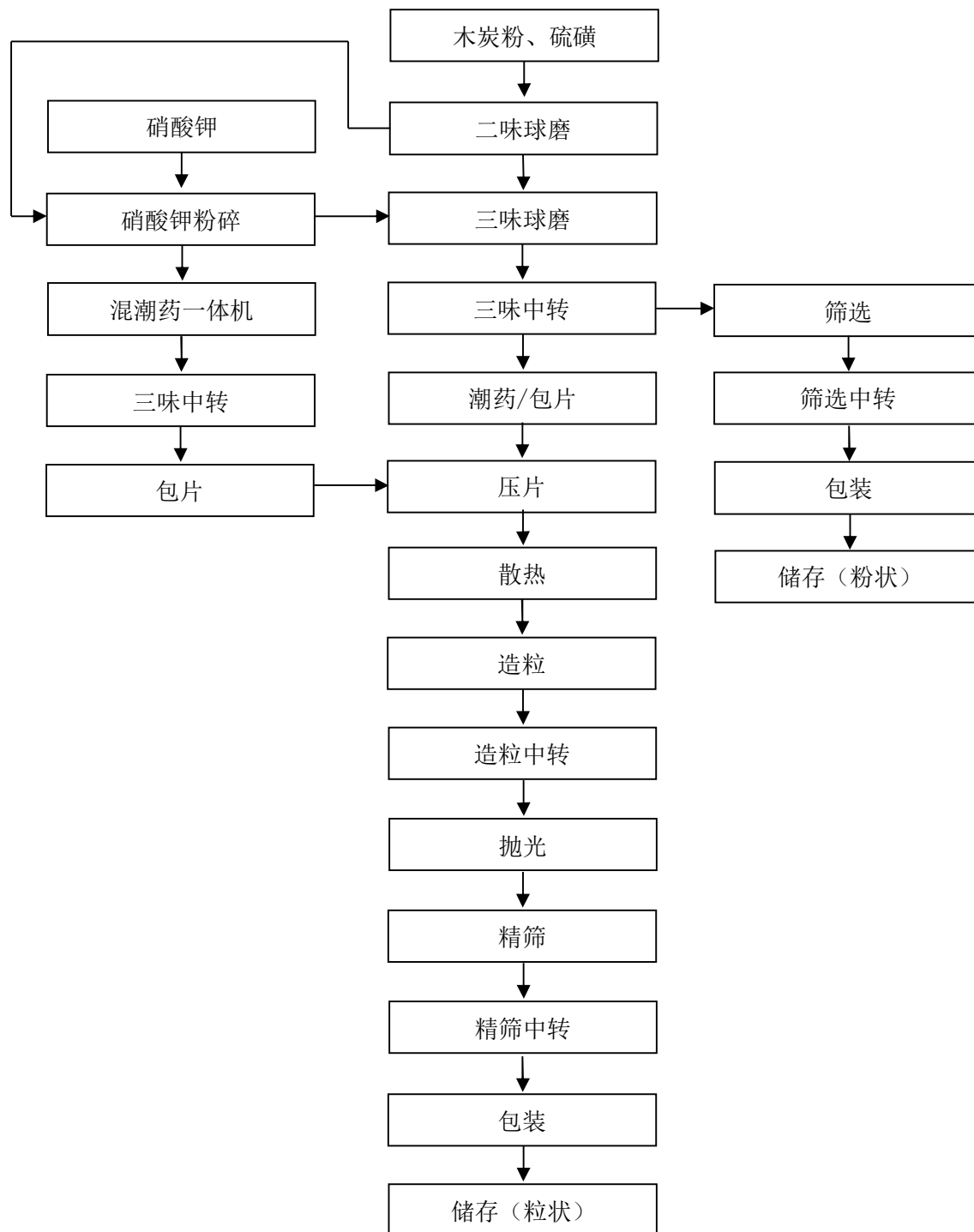
图 2.3-1 黑火药生产工艺流程图
