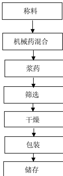
图 2-4-3 引药生产工艺流程图
