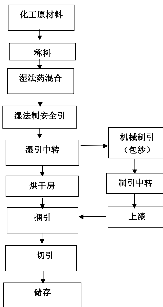
图 2-4-5 安全引（湿法）生产工艺流程
