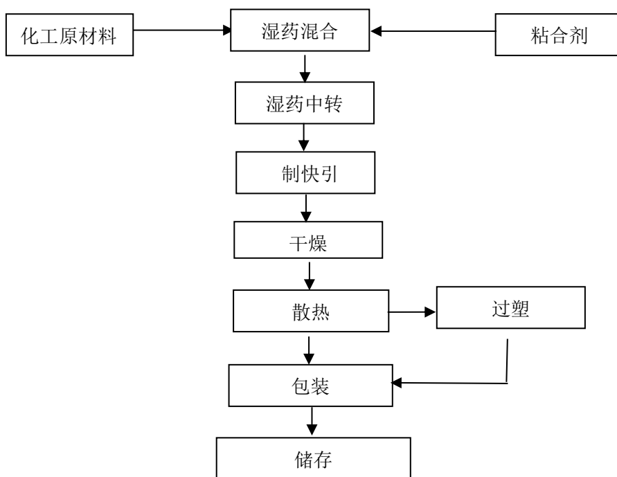
图 2-4-1 线引产品生产工艺流程图
