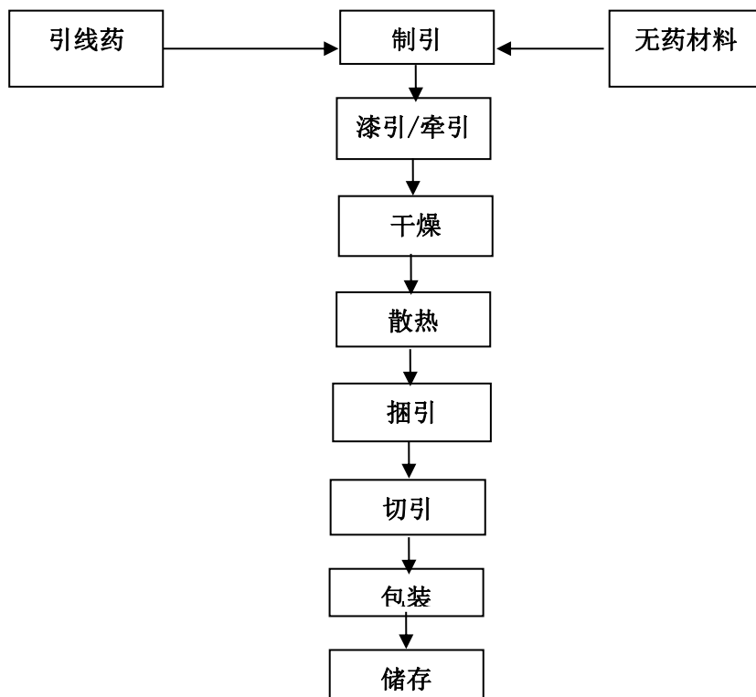
图 2-4-3 引药生产工艺流程图
