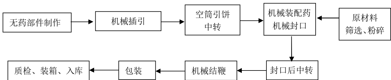
图 2-1：爆竹生产工艺流程图
