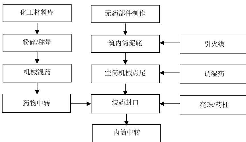
图 2.3-2：效果内筒生产工艺流程图
