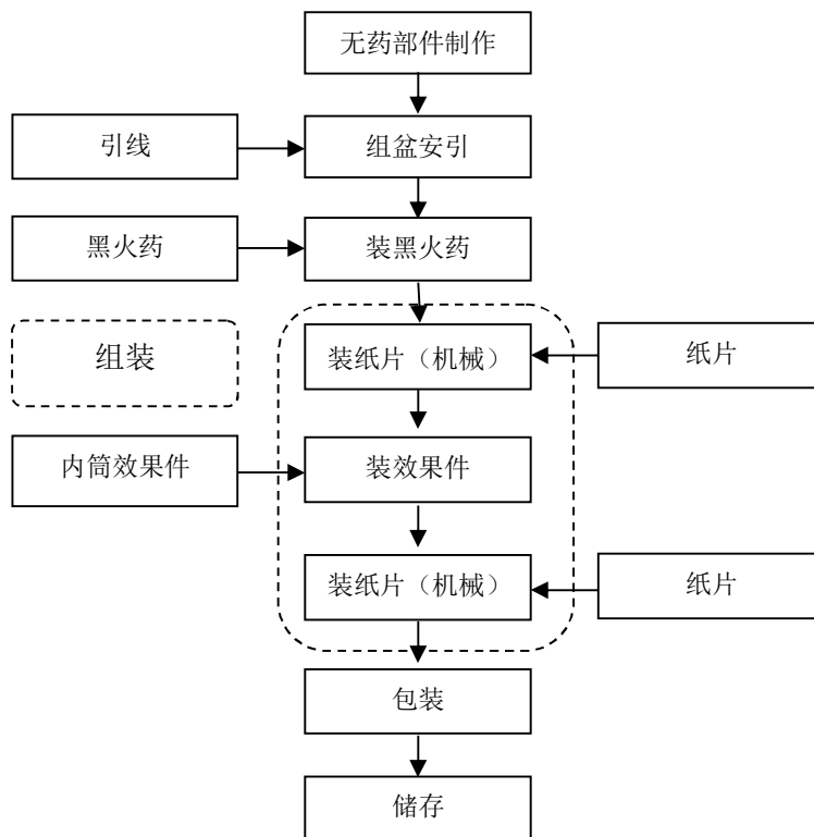
图 2.3-1：组合烟花生产工艺流程图
