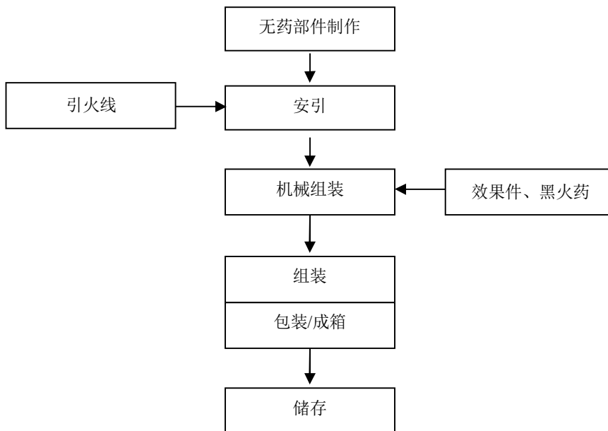
图 2.3-4：吐珠生产工艺流程图
