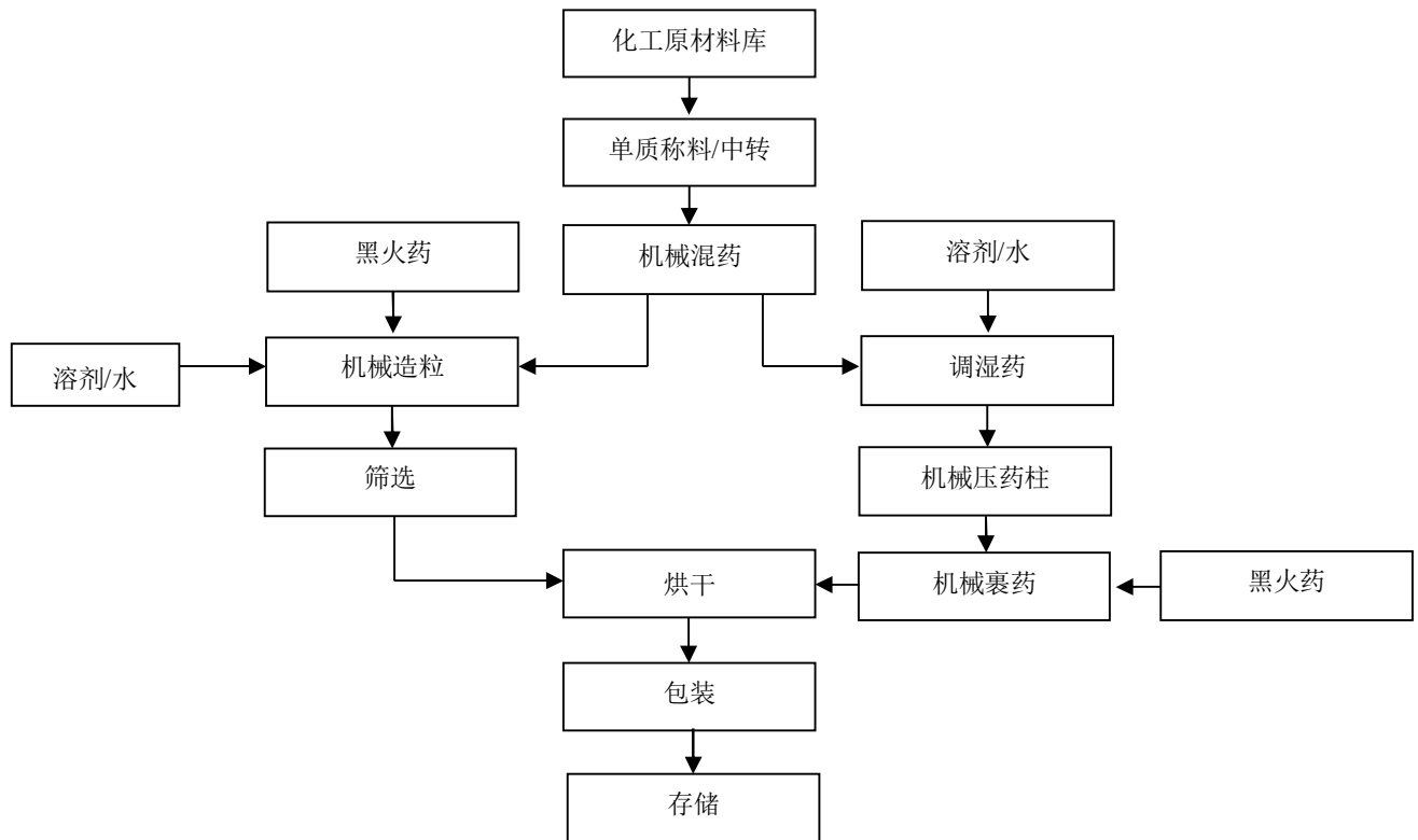
图 2.3-5：亮珠/药柱生产工艺流程图
