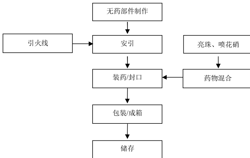
图 2.3-3：喷花生产工艺流程图
