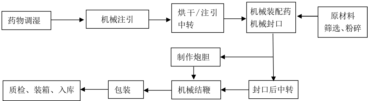
图 2-1：爆竹生产（注引）工艺流程图
