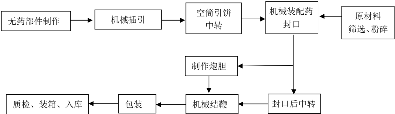
图 2-2：爆竹生产（插引）工艺流程图
