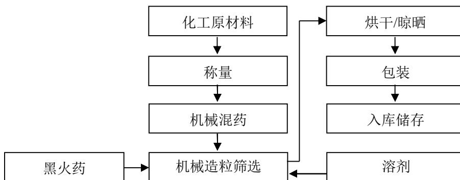
图 2.3-7：亮珠生产工艺流程图
