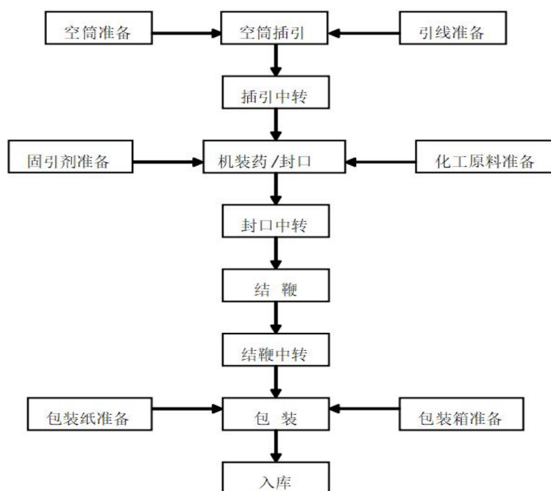
图 2-4-1 爆竹类产品生产工艺流程图
