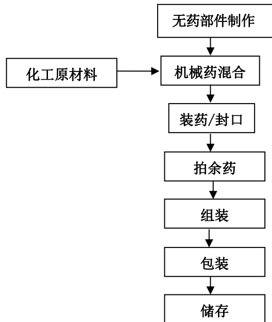
图 2-4-4 玩具类（线香型/晨光花）生产工艺流程图
