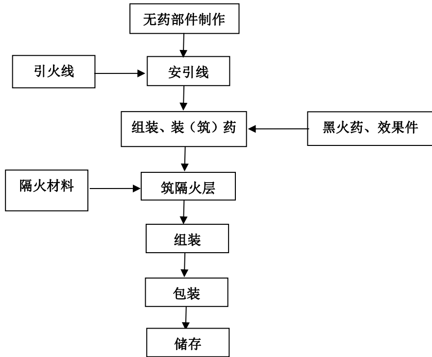
图 2-4-3 吐珠类产品生产工艺流程图
