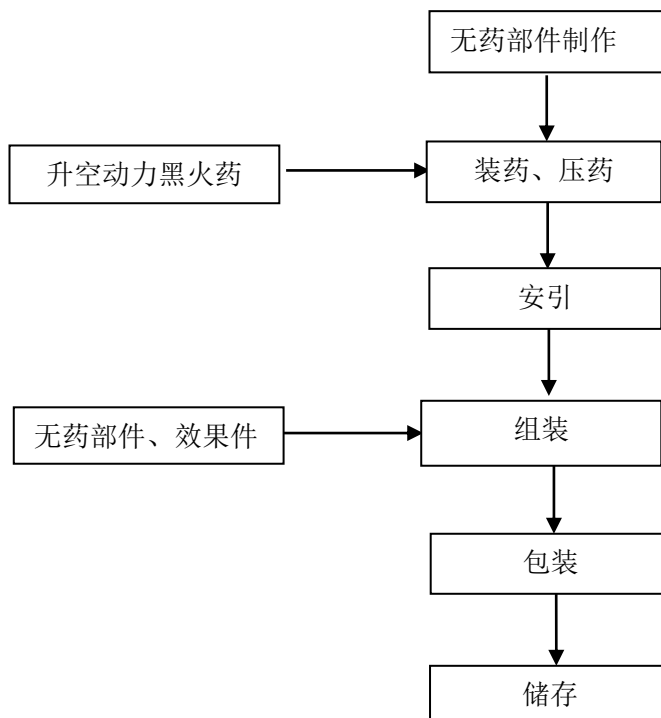
图 2.4-7 升空类（火箭）产品生产工艺流程图
