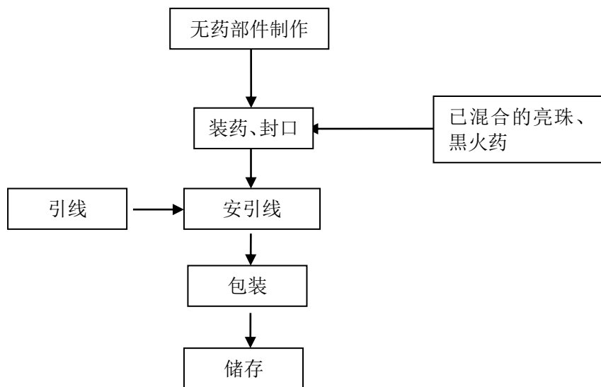
图 2.4-3 喷花类产品生产流程图
