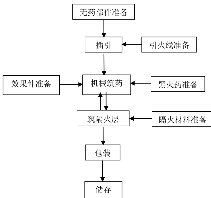
图 2.4-1 吐珠类产品生产工艺流程图
