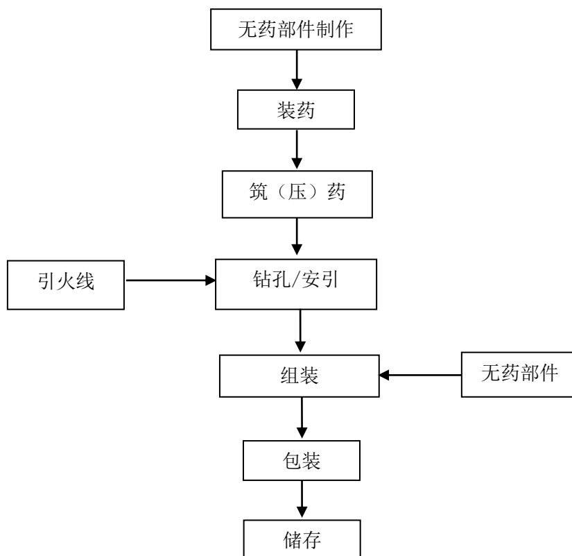
图 2.4-4 旋转升空类生产工艺流程图
