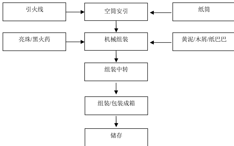
图 2-1：吐珠类生产工艺流程图
