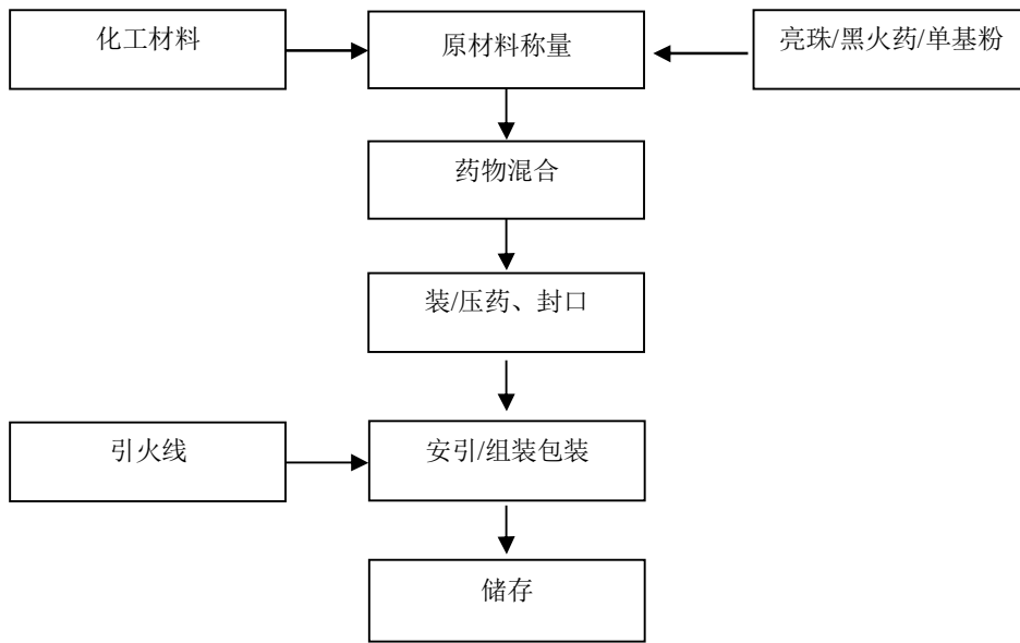
图 2-2：喷花类生产工艺流程图
