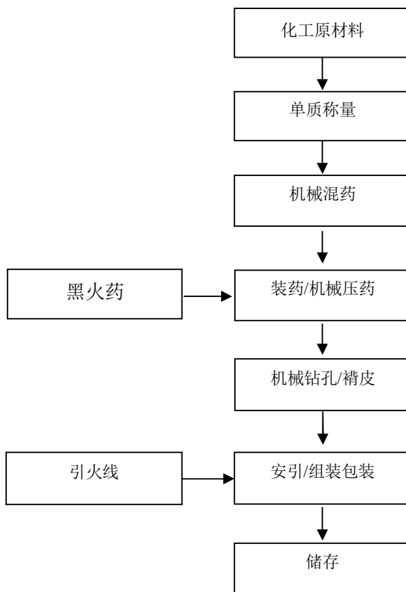
图 2-3：升空类（旋转升空烟花）/旋转类（大地花开）生产工艺流程图
