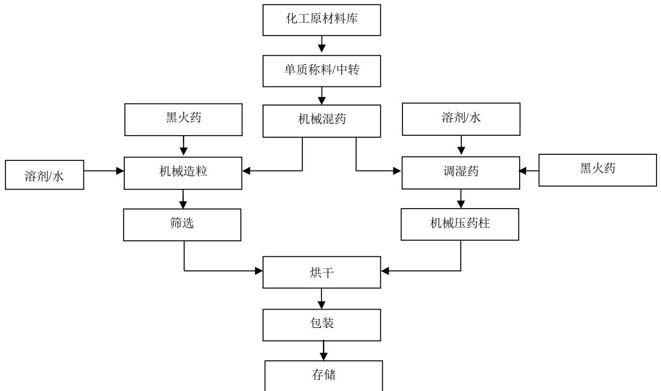
图 2-4：亮珠/药柱生产工艺流程图
