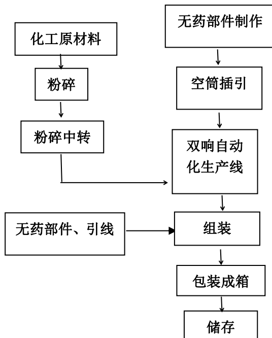
图 2-4-1 升空类（双响炮）生产流程图
