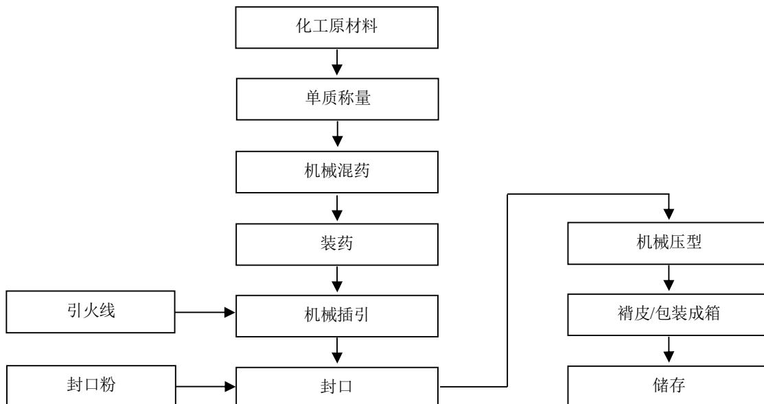
图 2-5：旋转类（彩菊）生产工艺流程图
