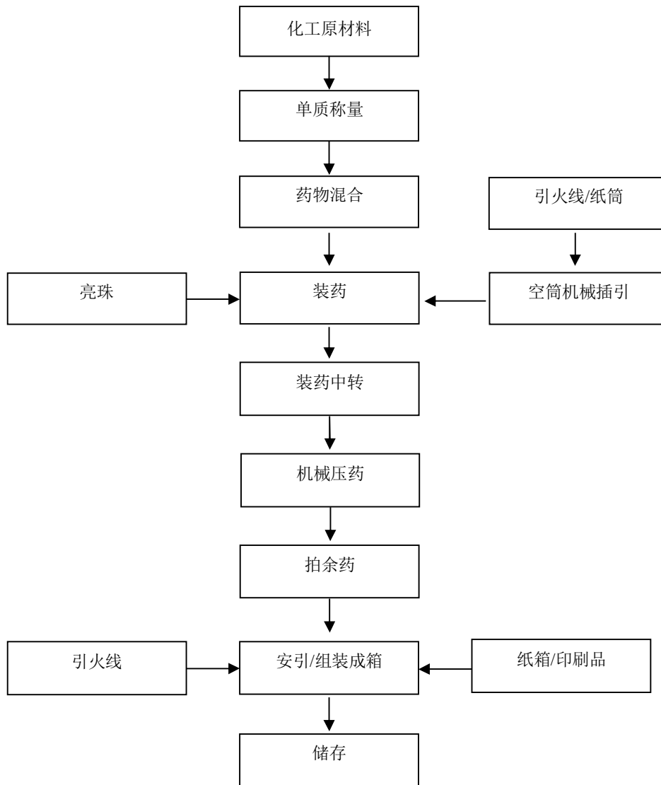
图 2-1：升空类（火箭）生产工艺流程图
