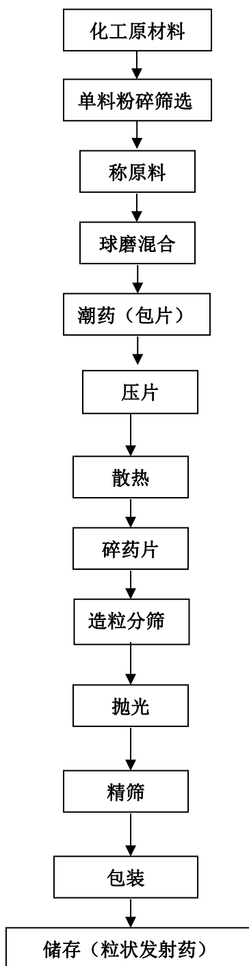
黑火药制造工艺流程图
