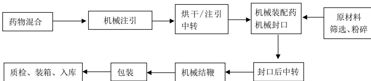
图 2-2: 爆竹生产 (注引) 工艺流程图
