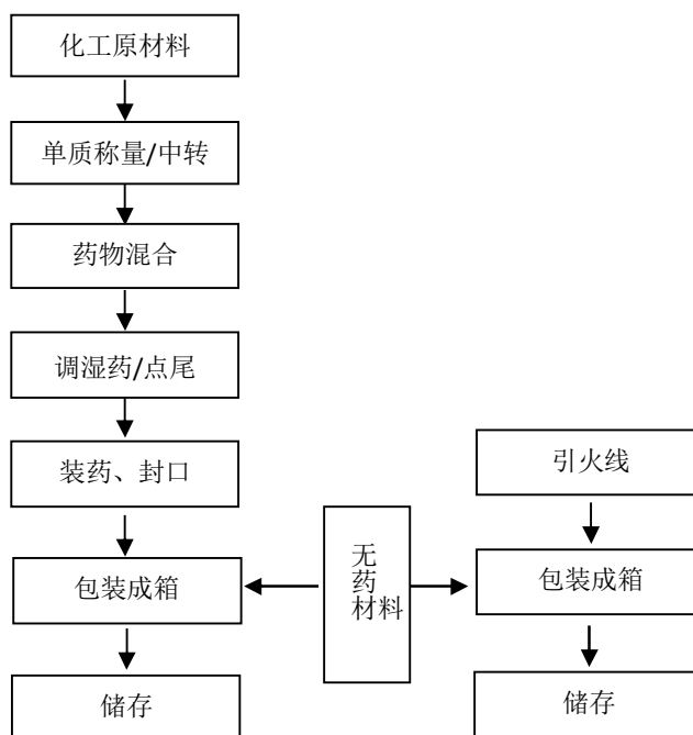
图 2-3: 玩具类 (线香型-晨光花) 生产工艺流程图
