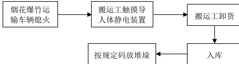
图 2-2-2-1 烟花爆竹入库工艺流程示意图
