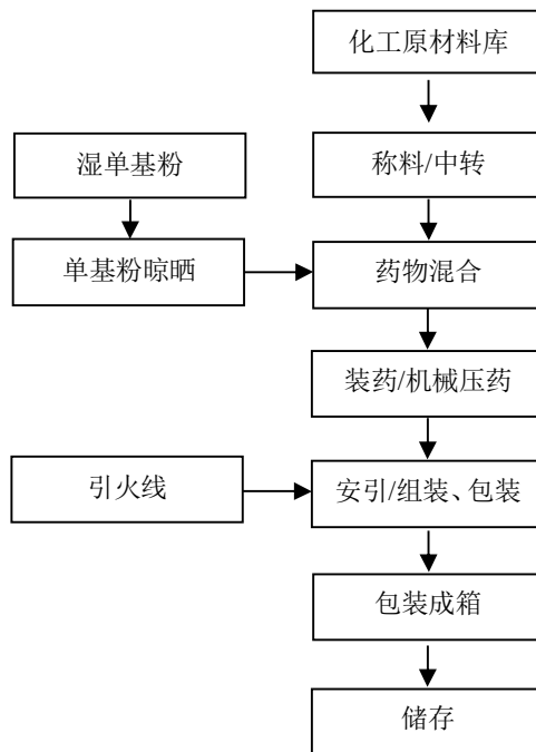
图 2-5：玩具类（玩具造型）生产工艺流程图
