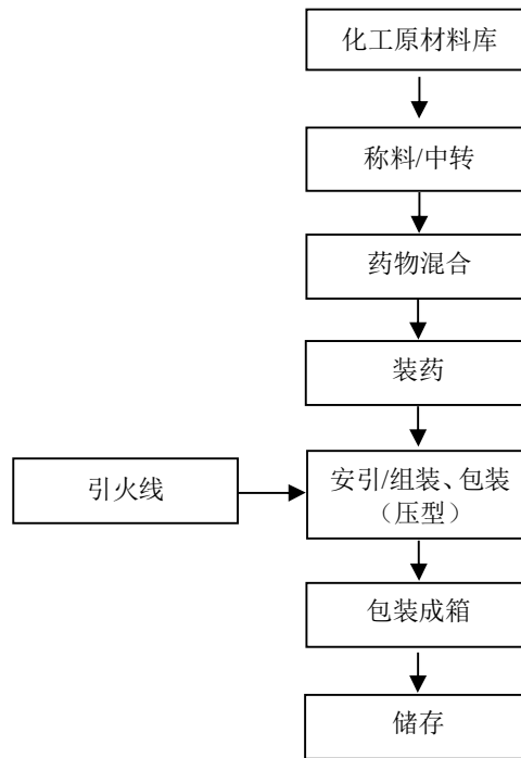
图 2-6：旋转类（有轴）生产工艺流程图
