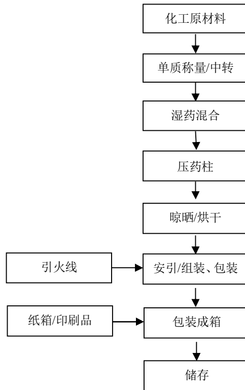
图 2-4：玩具类（烟雾型）生产工艺流程图
