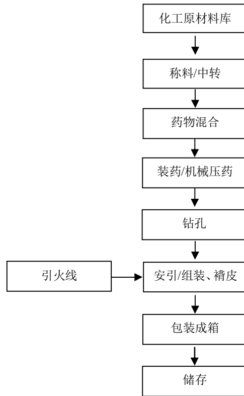
图 2-8: 升空类（旋转升空）生产工艺流程图
