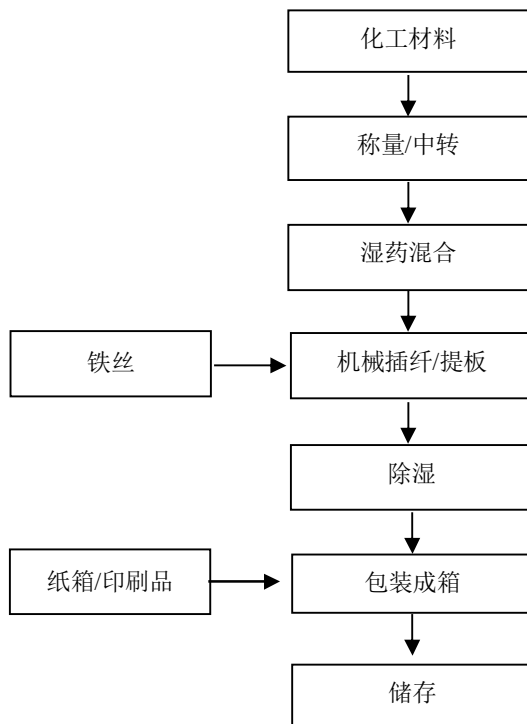
图 2-3: 玩具类（线香型—电光花）生产工艺流程图
