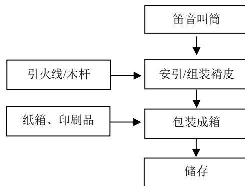
图 2-9: 升空类（火箭）生产工艺流程图
