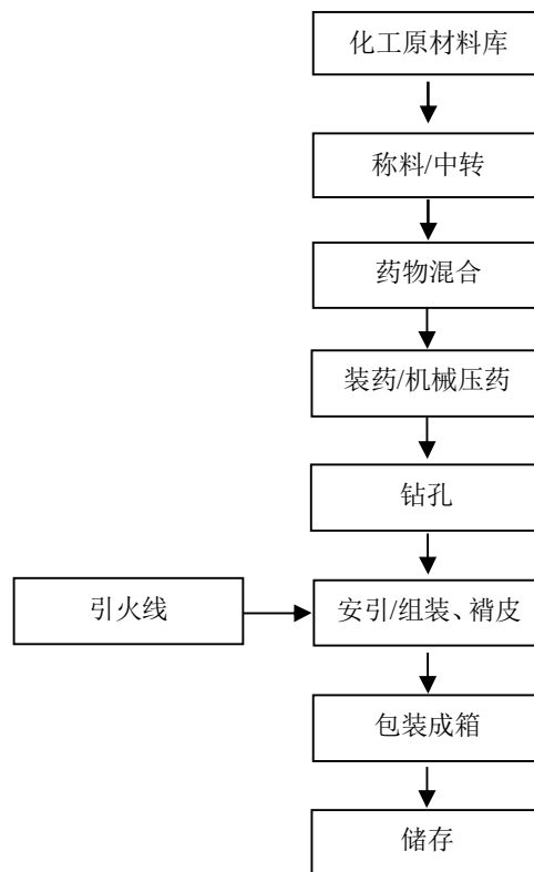
图 2-7：旋转类（无轴）生产工艺流程图
