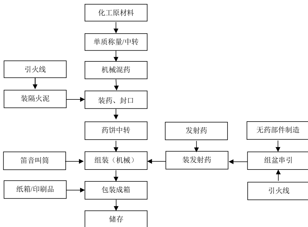
图 2-1：组合烟花类（不含亮珠）生产工艺流程图
