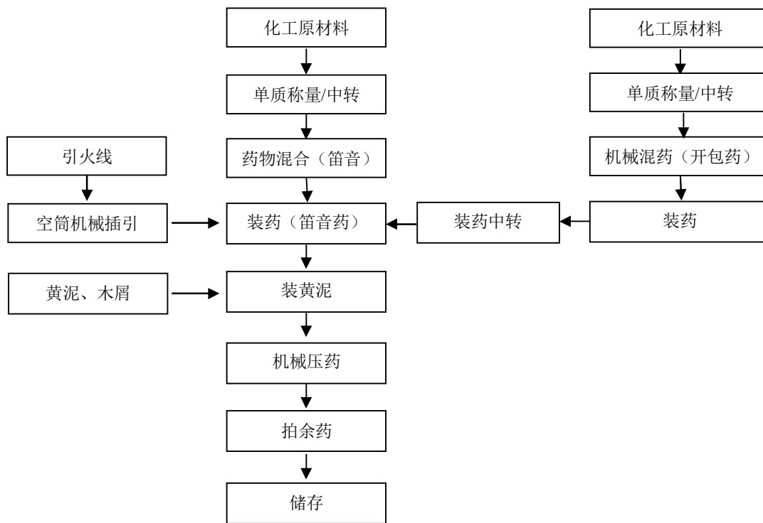
图 2-2: 笛音叫筒生产工艺流程图
