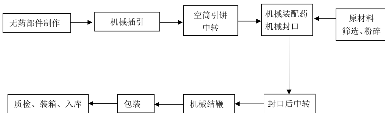
图 2-1：爆竹生产（插引）工艺流程图
