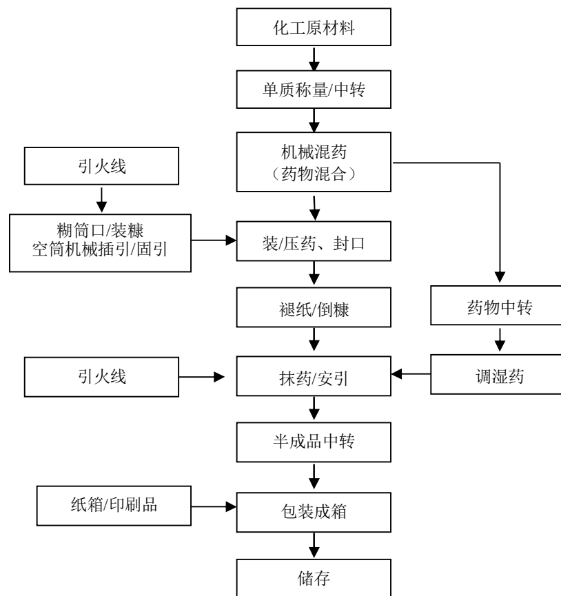
图 2-2：喷花类（闪光炮）生产工艺流程图
