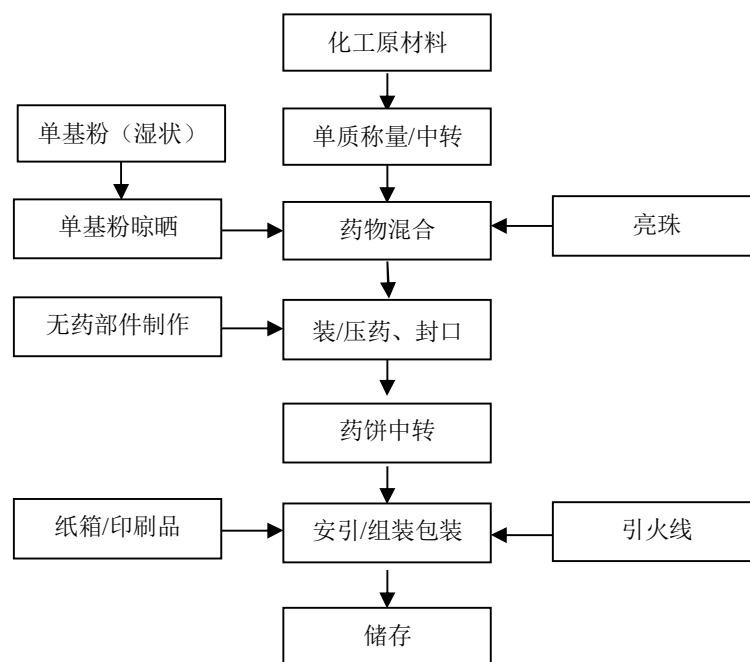
图 2-1：喷花类（喷花）生产工艺流程图
