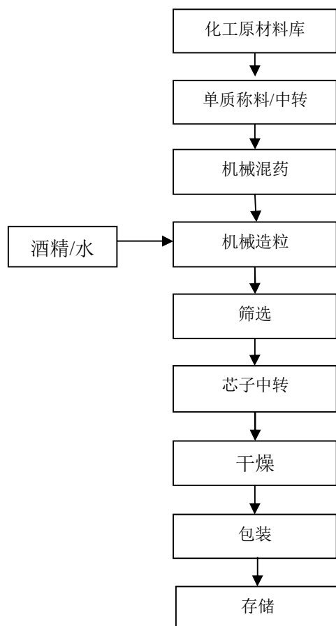
图 2-6：亮珠生产工艺流程图
