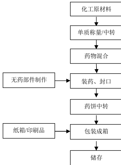
图 2-4：玩具类（线香型—晨光花）生产工艺流程图
