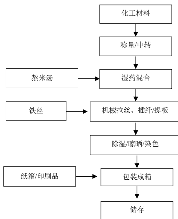
图 2-3：玩具类（线香型—电光花）生产工艺流程图
