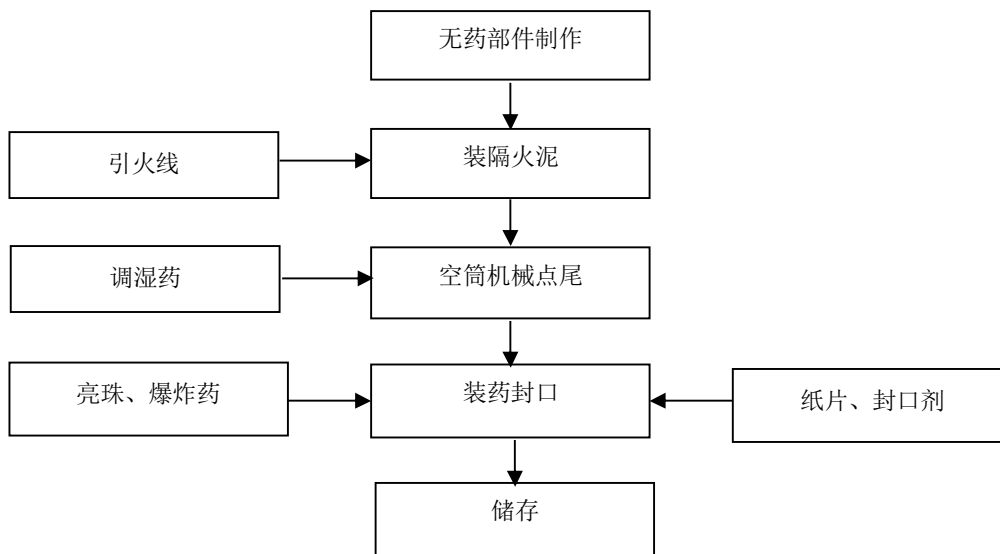
图 2-2: 效果内筒（柱形）生产工艺流程图
