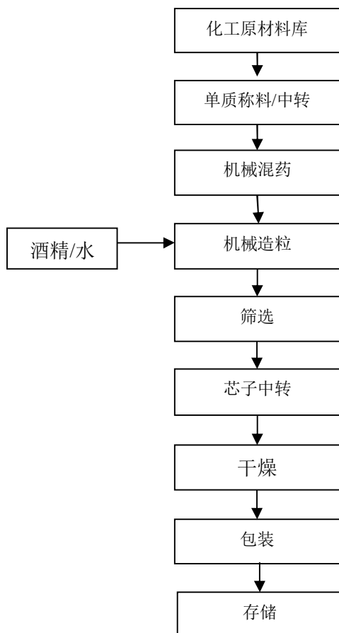
图 2-7: 亮珠生产工艺流程图
