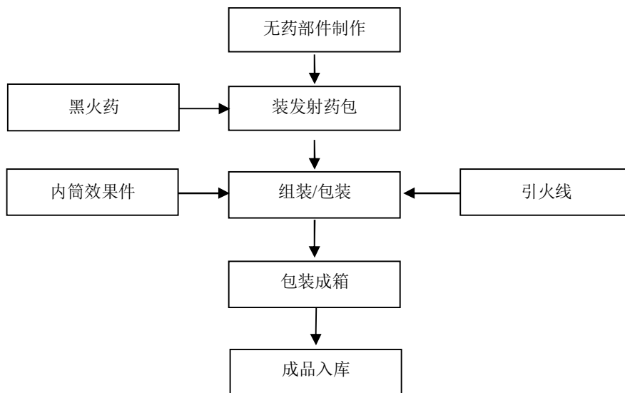
图 2-4：小礼花生产工艺流程图
