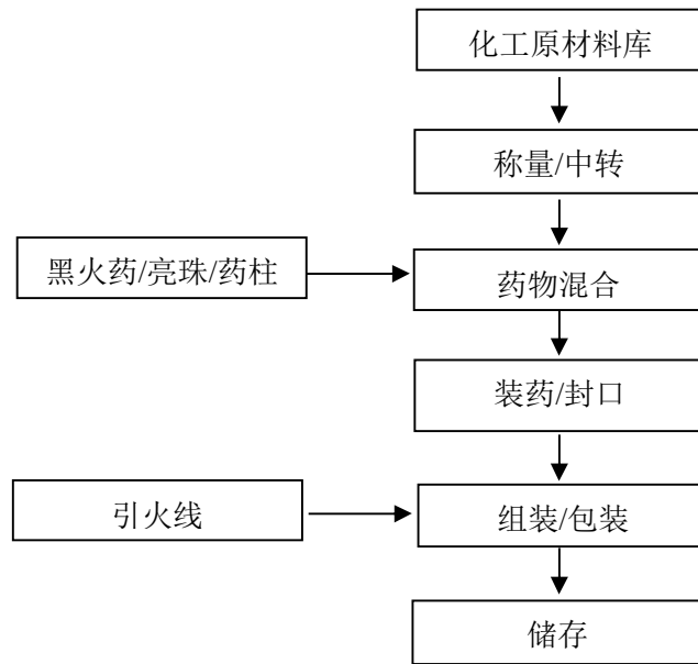
图 2-6: 喷花类/玩具类产品生产工艺流程图
