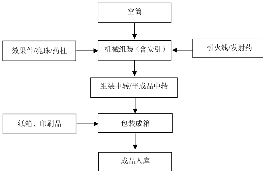
图 2-5：吐珠类产品生产工艺流程图
