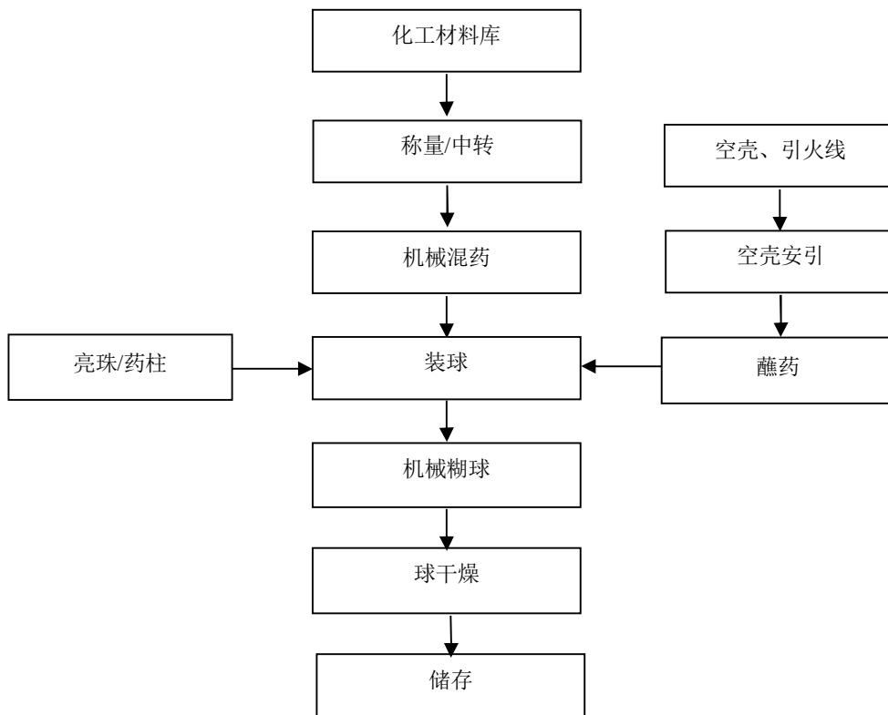
图 2-3: 效果内筒（球型）生产工艺流程图
