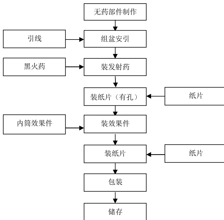
图 2-1：组合烟花生产工艺流程图
