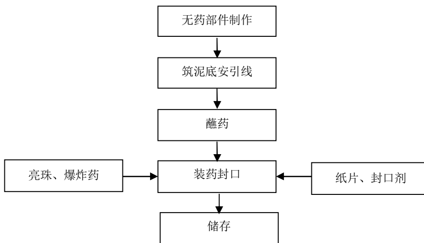
图 2-2：效果内筒生产工艺流程图
