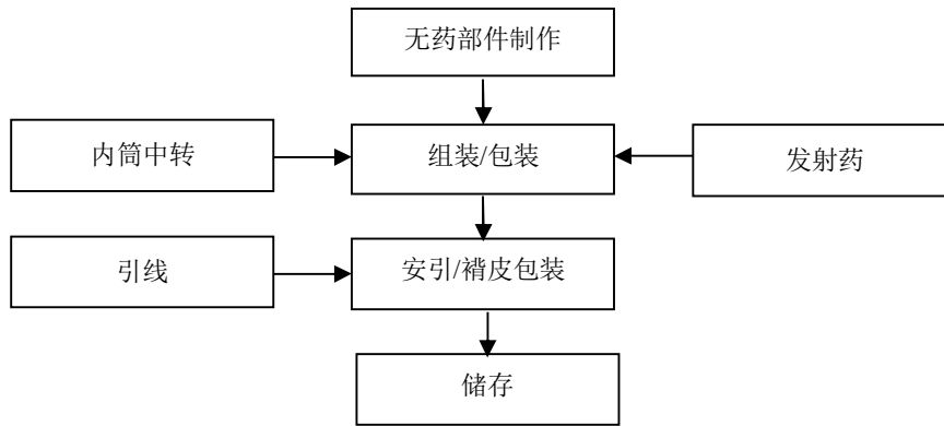
图 2-3：小礼花生产工艺流程图
