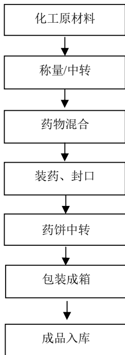
图 2-7：线香型生产工艺流程图
