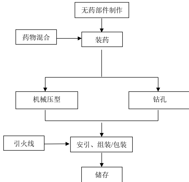
图 2-4：旋转类产品生产工艺流程图
