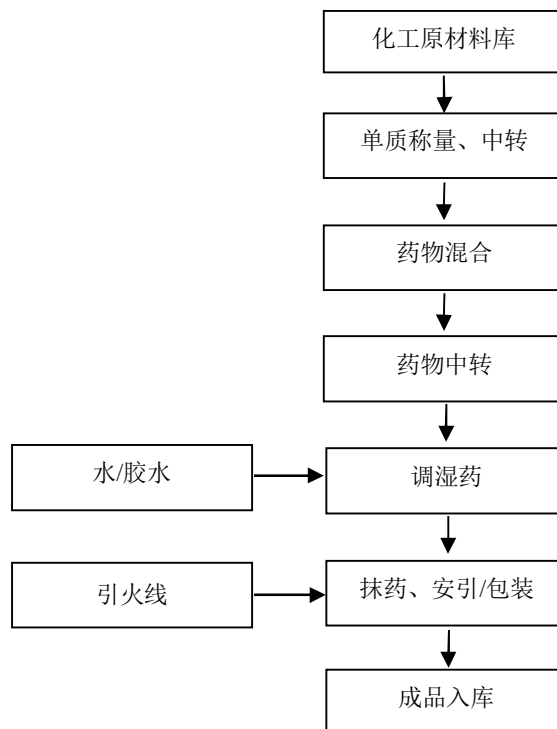
图 2-5：喷花类产品（闪光）生产工艺流程图
