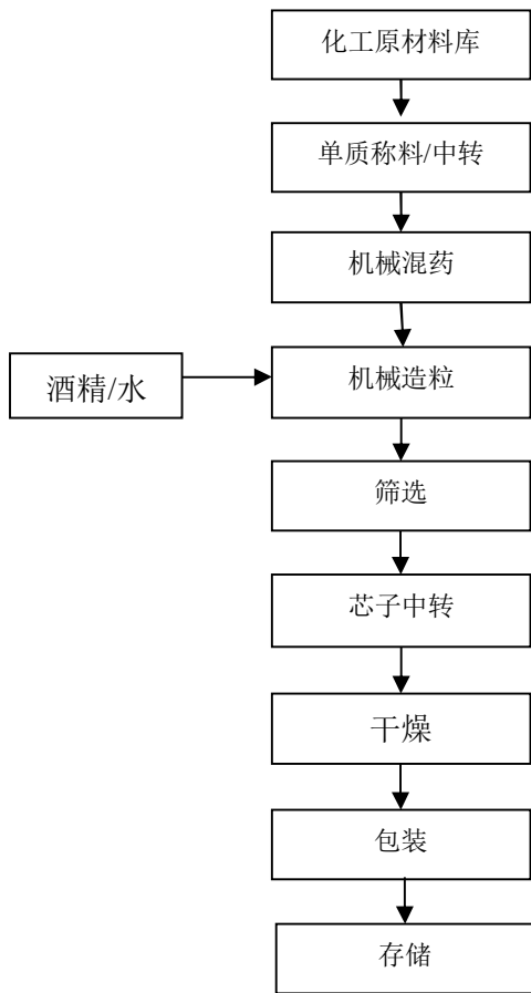
图 2-9: 亮珠生产工艺流程图
