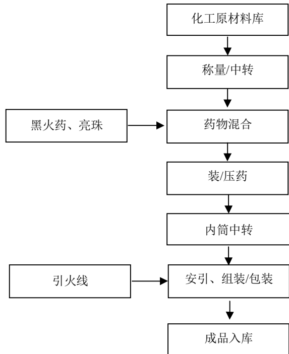
图 2-8：玩具造型生产工艺流程图
