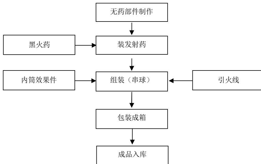
图 2-3: 小礼花生产工艺流程图
