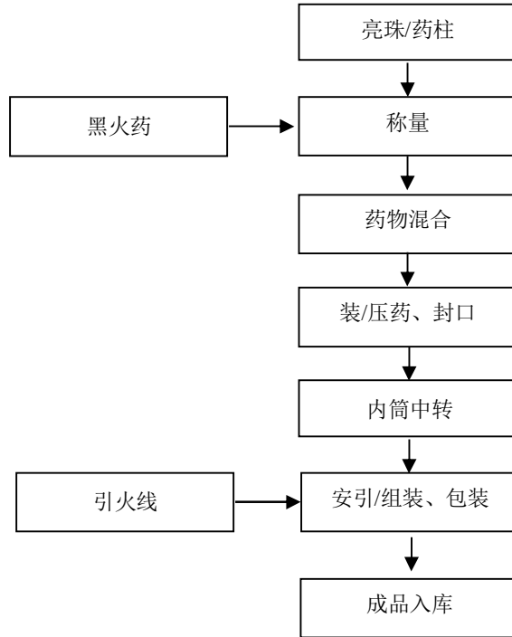
图 2-6：喷花类产品（花筒）生产工艺流程图
