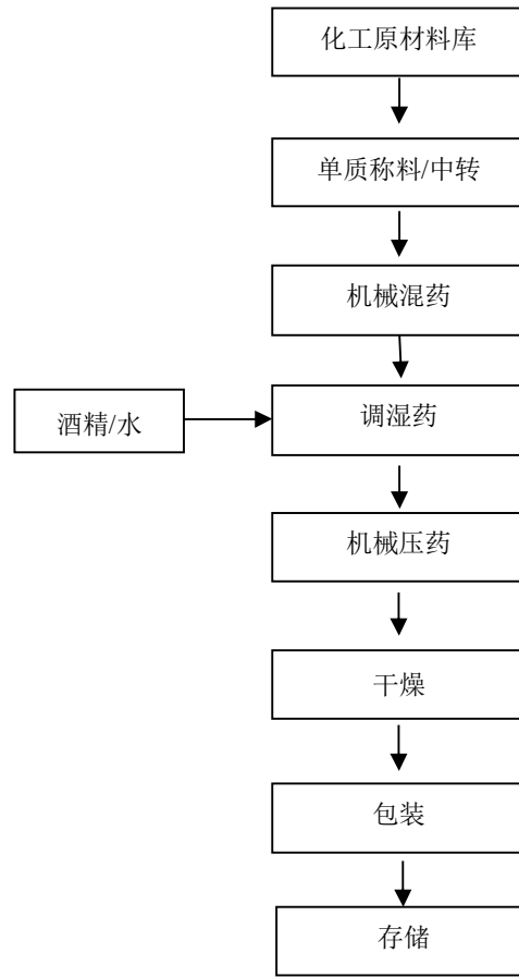
图 2-10: 药柱生产工艺流程图
