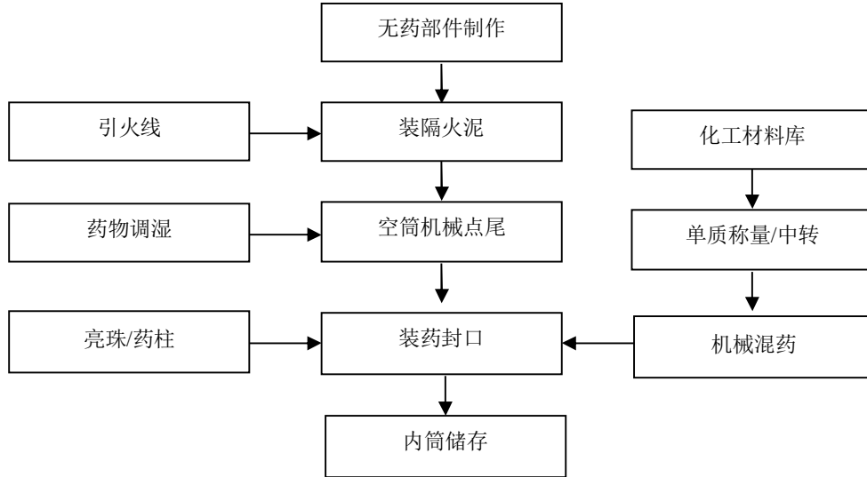
图 2-2: 柱型效果内筒生产工艺流程图
