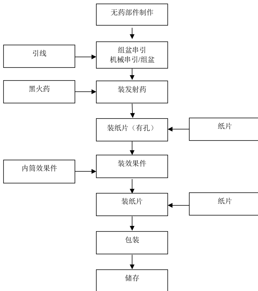
图 2-1：组合烟花生产工艺流程图
