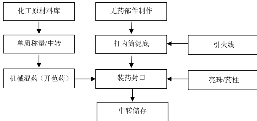
图 2-2: 效果内筒（柱型）生产工艺流程图
